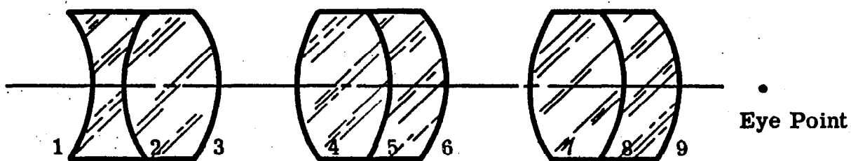
ERFLE EYEPIECE
