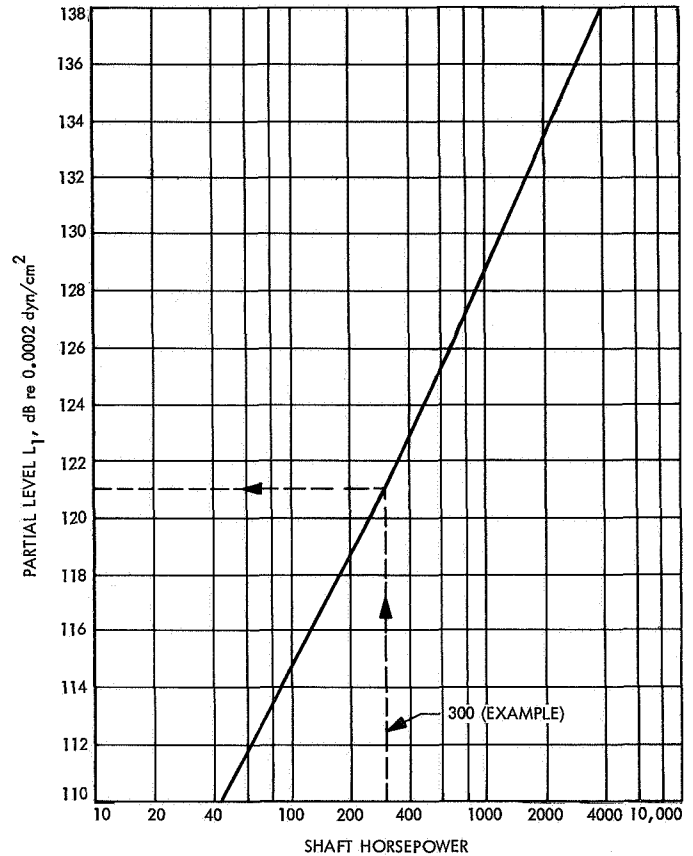
Fig. B-2. Reference level
