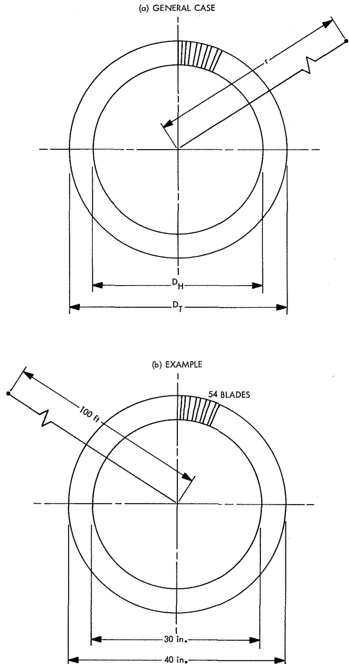
Fig. D-1. Lift fan axis system
