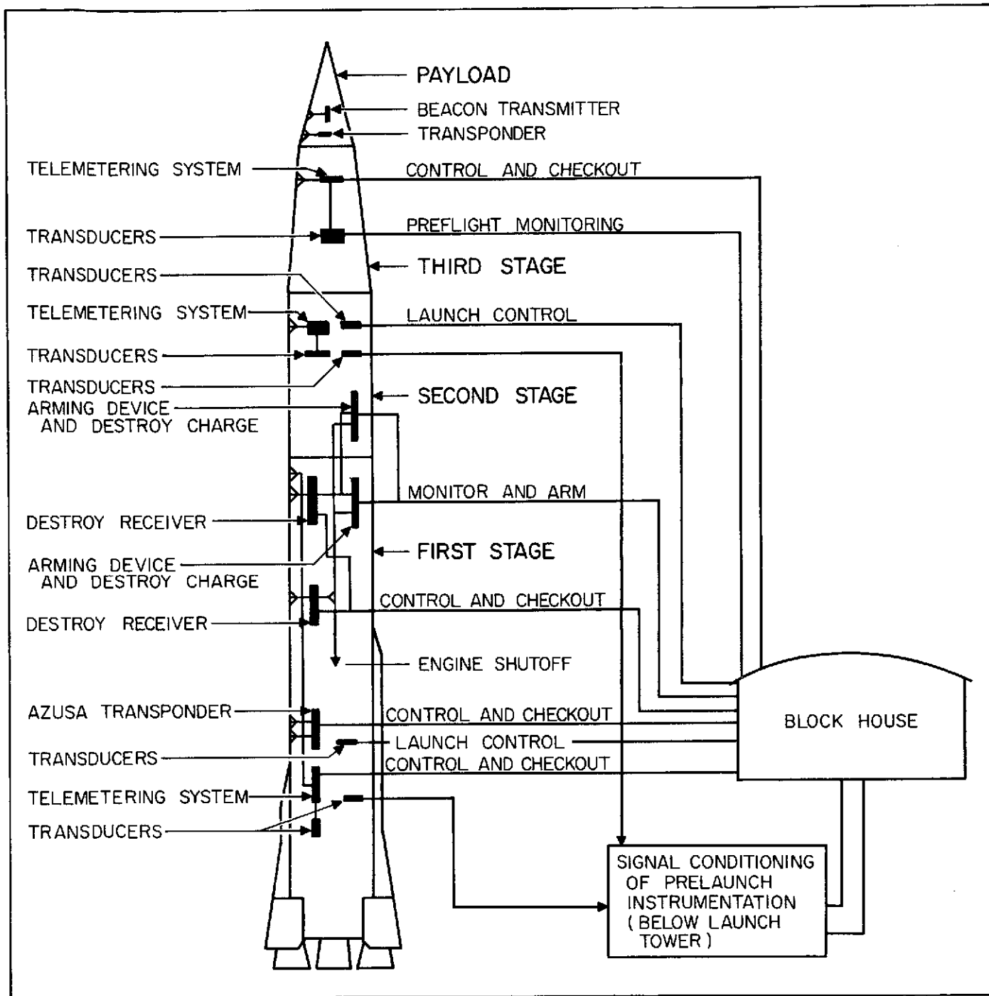
Fig. 17. Vega Airborne Instrumentation
