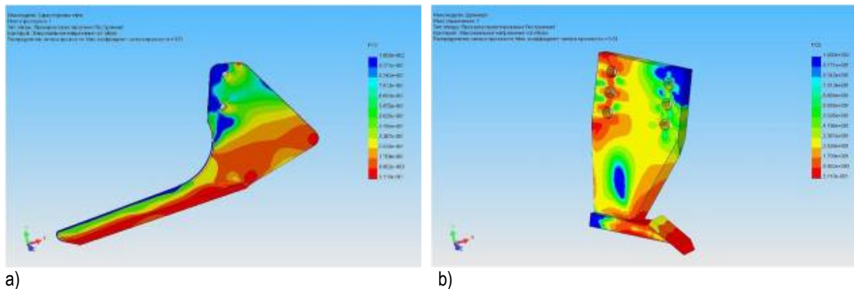
a) b) Figure 7 : Répartition des champs de contraintes sur les surfaces des socs unilatéraux (a) et des dents de la sous-soleuse (b).
