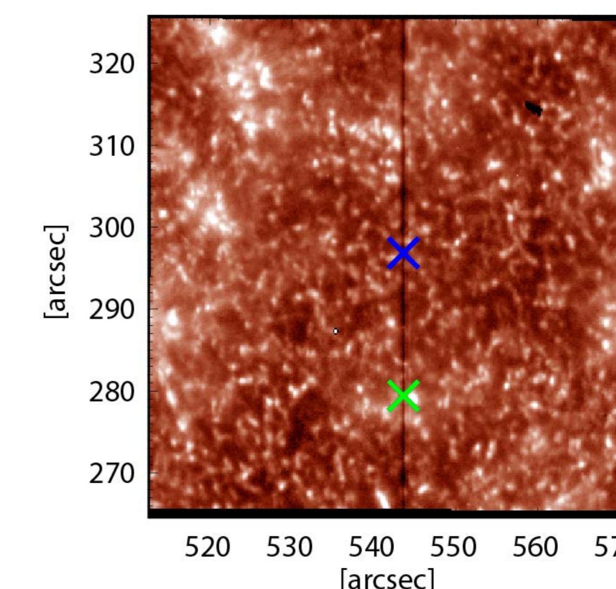
Fig.3 IRIS SJI (1400)
