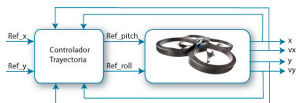
Figura 2: Bloque de control para el CIC2012. Los participantes, a partir de posición y velocidad, obtuvieron un modelo y desarrollaron un controlador para seguimiento de trayectorias.
