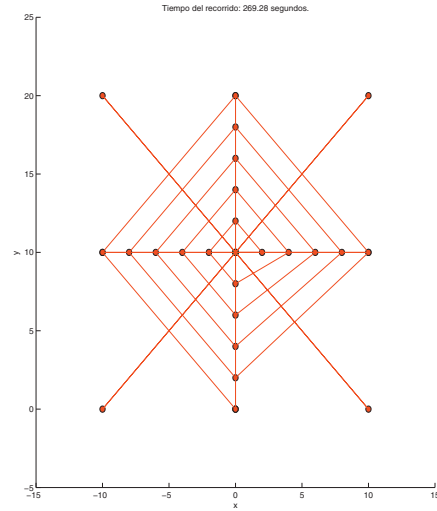
Figura 5: Trayectoria empleada para la evaluación del controlador.
