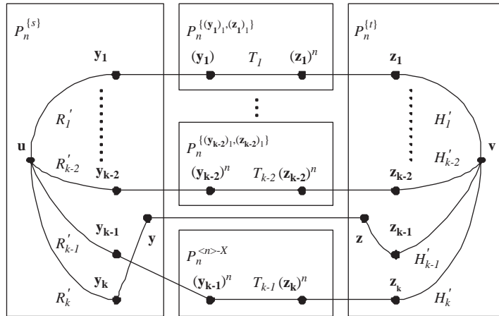
Fig. 3. Illustration for Lemma 5.
