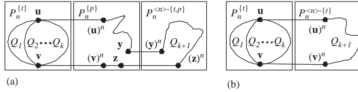
Fig. 2. Illustration for Lemma 4.
