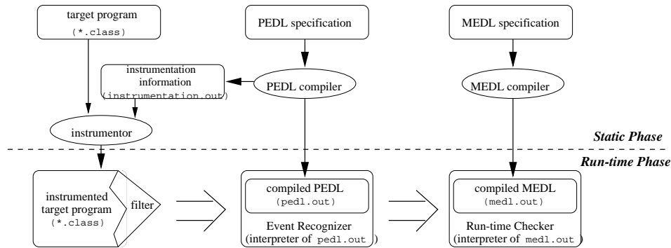
Fig. 6. Java-MaC
