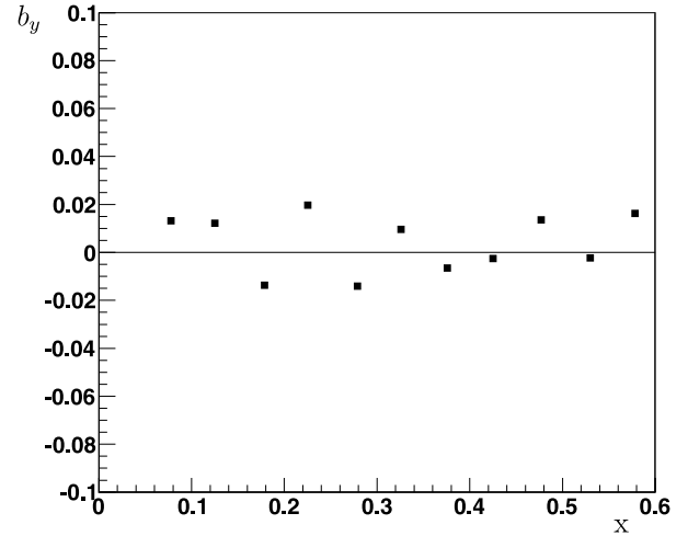
Fig. 10. Extra shift b_y vs x .
