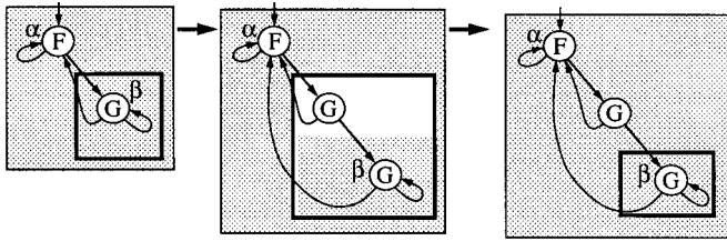
FIG. 26. Analysis of \mu -step.
