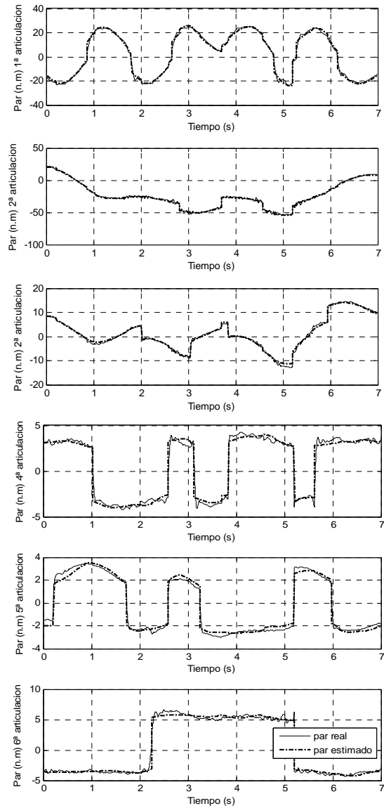
Figura 2. Pares medidos y calculados del robot PUMA.
