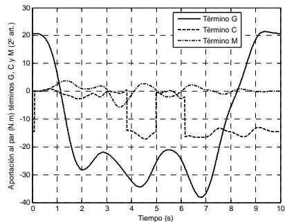
Figura 9. Aportación términos dinámicos de gravedad, Coriolis e inerciales al par de la 2ª articulación del PUMA.
