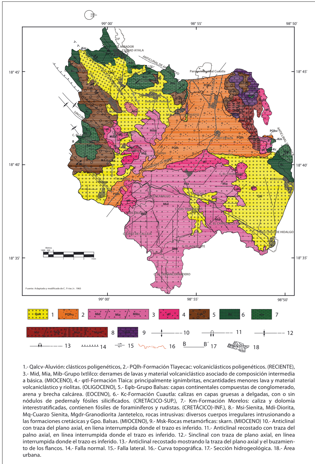
Figura 2. Mapa geológico de la región de Tenextepango, Morelos. Fuente: Varela (2011).
