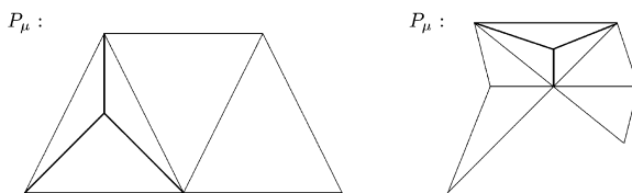
Fig. 2. Subdivision of a triangle.
