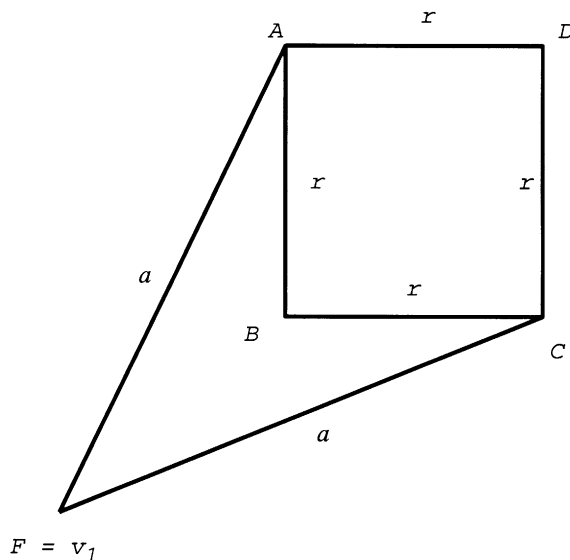
Fig. 10. The Peaucellier inversor.
