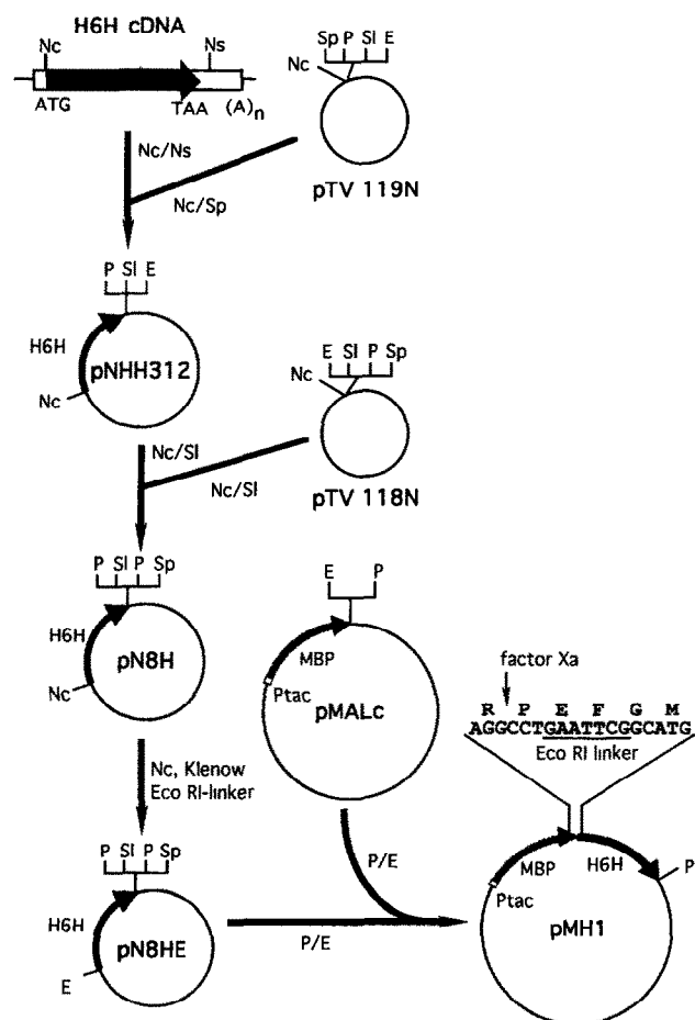
Fig. 2. Construction of the H6H expression vector pMH1. E, EcoRI ; Nc, NcoI ; Ns, NspI ; P, PstI ; SI, Sall ; Sp, SphI .
