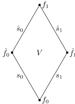
Fig. 1. A Bianchi quadrilateral.
