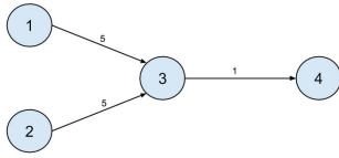
Fig. 1. The actorsystem
