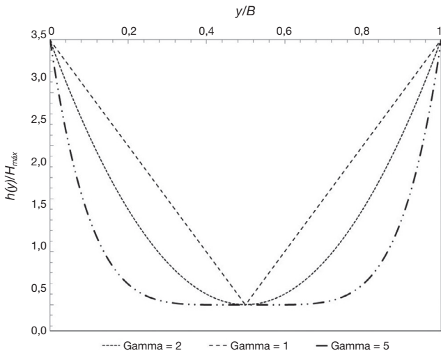
Figura 4. Distribuciones transversales de profundidades obtenidas utilizando distintos valores del parámetro \gamma en la ecuación 3.
