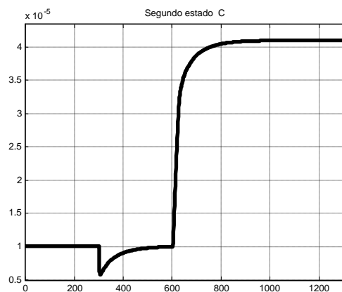
Figura 5. Respuesta del segundo estado ( C ) ante la perturbación aplicada.
