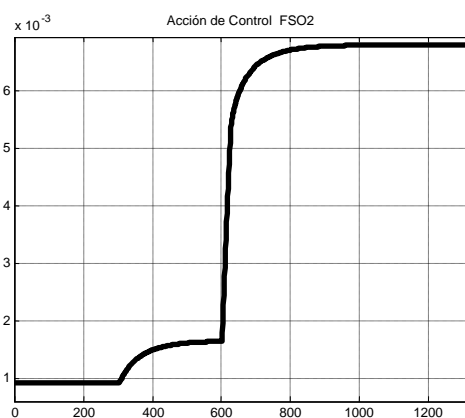
Figura 6. Comportamiento de la acción de control (Flujo de humos F_2 ) en respuesta a la perturbación aplicada.
