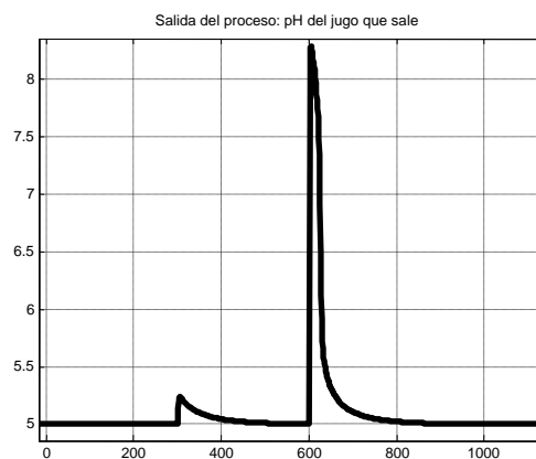
Figura 7. pH de salida de la sulfitadora ante la perturbación aplicada.
