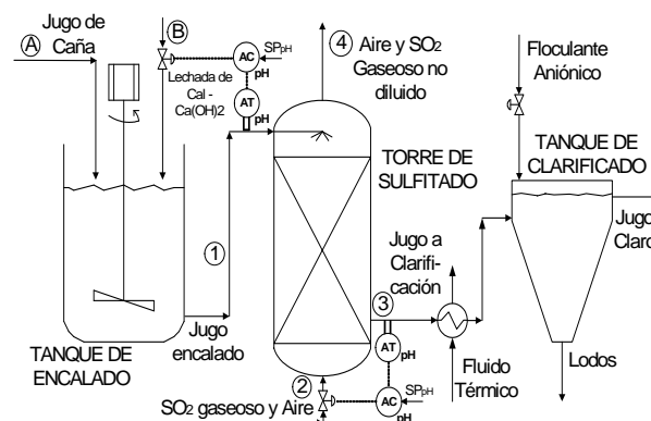
Figura 1. Diagrama de flujo general para el proceso de clarificación.
