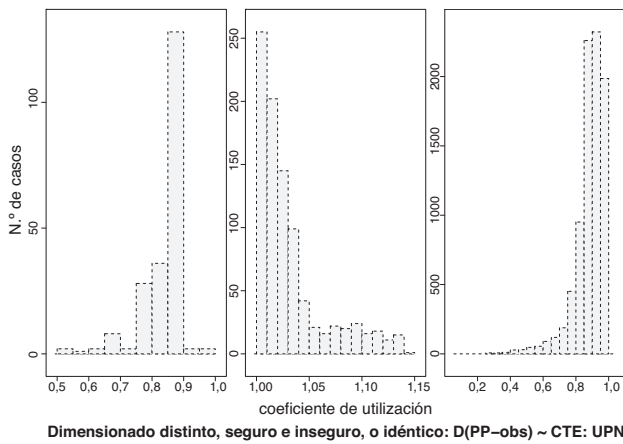
Figura 6. Dimensionado PP-obs, con UPN en cajón.
