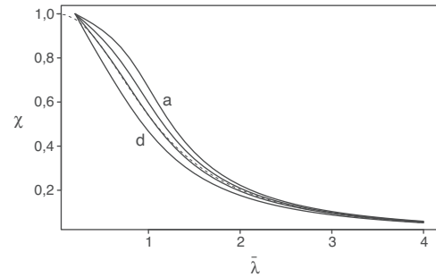
Figura 1. Curvas de pandeo a, b, c, d, y aproximación.
