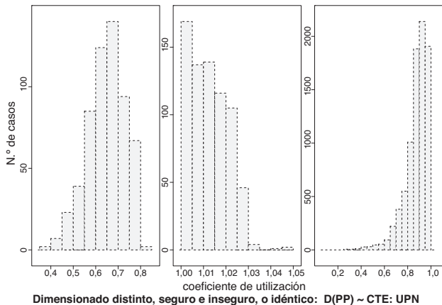
Figura 7. Dimensionado propuesto en este texto: caso UPN PP.
