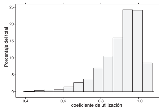
Figura 12. Dimensionado aproximado: \kappa Center exacto para los tubos empleados.
