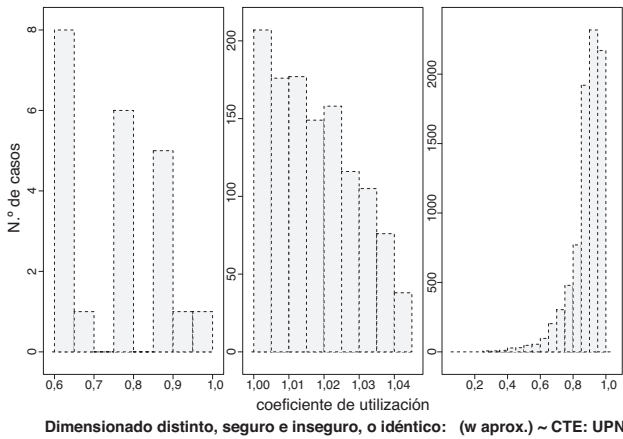
Figura 5. Aproximación con \omega(\lambda) \approx 1 + (\lambda/100)^3 : caso UPN \omega -obs.
