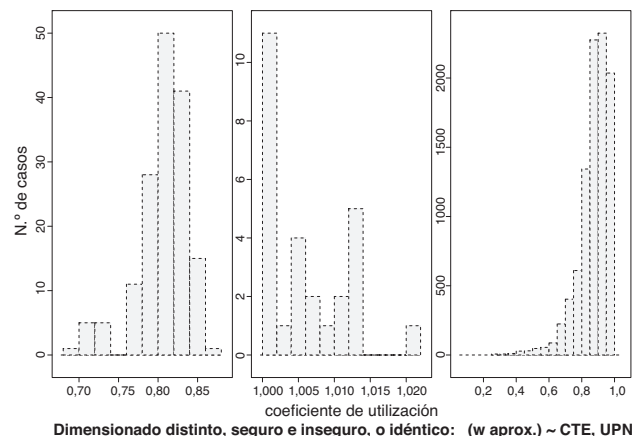
Figura 4. Aproximación con \omega(\lambda) \approx 1 + (\lambda/\lambda_{w=2})^{2,2} : caso UPN \omega -ap.
