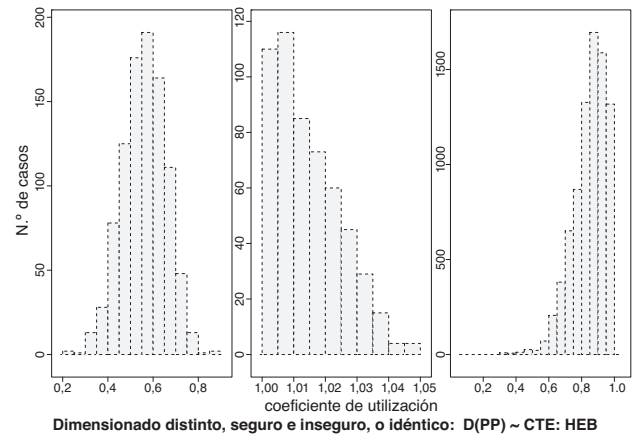
Figura 8. Dimensionado propuesto en este texto: caso HEB PP.
