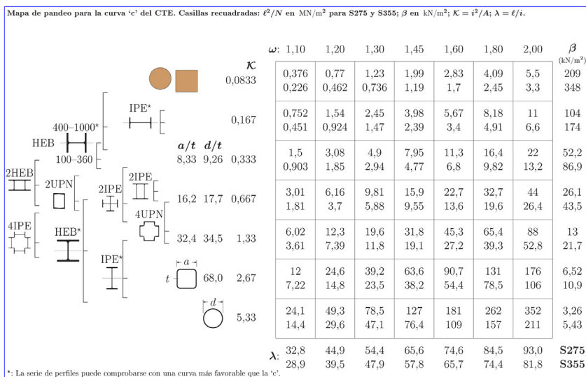
Figura 16. Mapa de pandeo para la curva 'c' del CTE.
