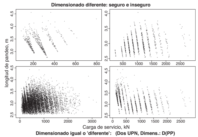
Figura 10. Dimensionado aproximado propuesto: casos de carga y altura.
