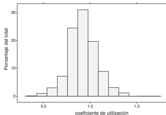
Figura 11. Dimensionado aproximado: \kappa estimada en gama de perfiles «20».
