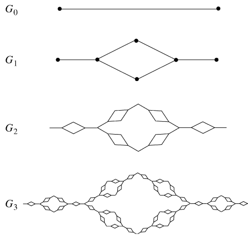
Fig. 1. The Laakso graphs.
