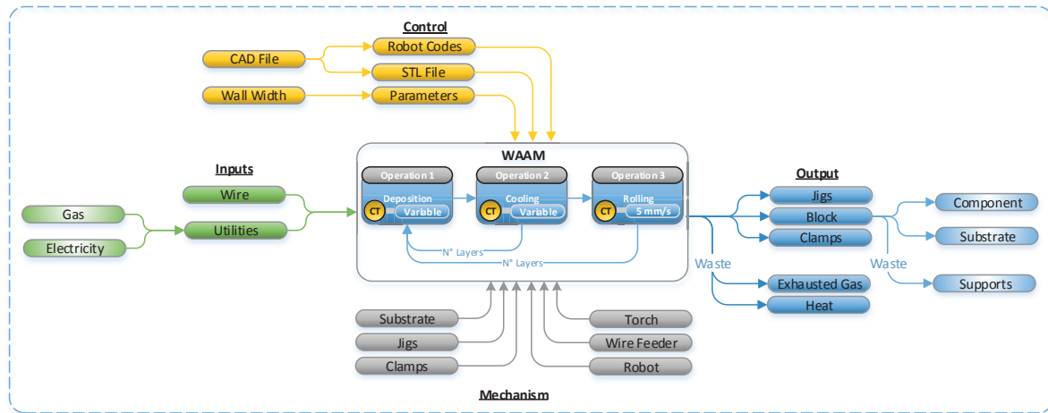
Fig. 3. - WAAM IDEF0
