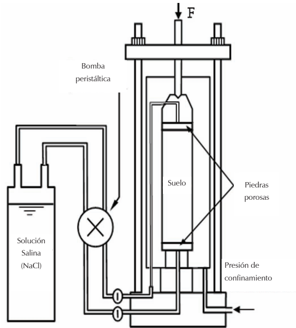
Figura 2. Aparato triaxial con succión controlada
