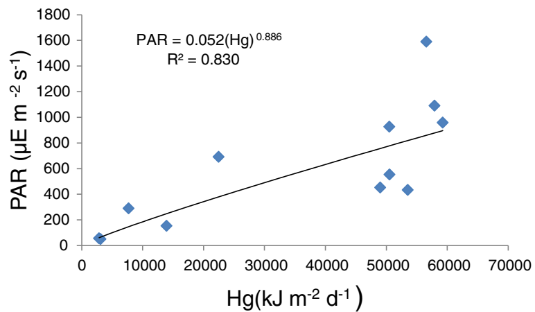
Figure 6 Estimated PAR vs Hg ( \Phi = 29^\circ ).
