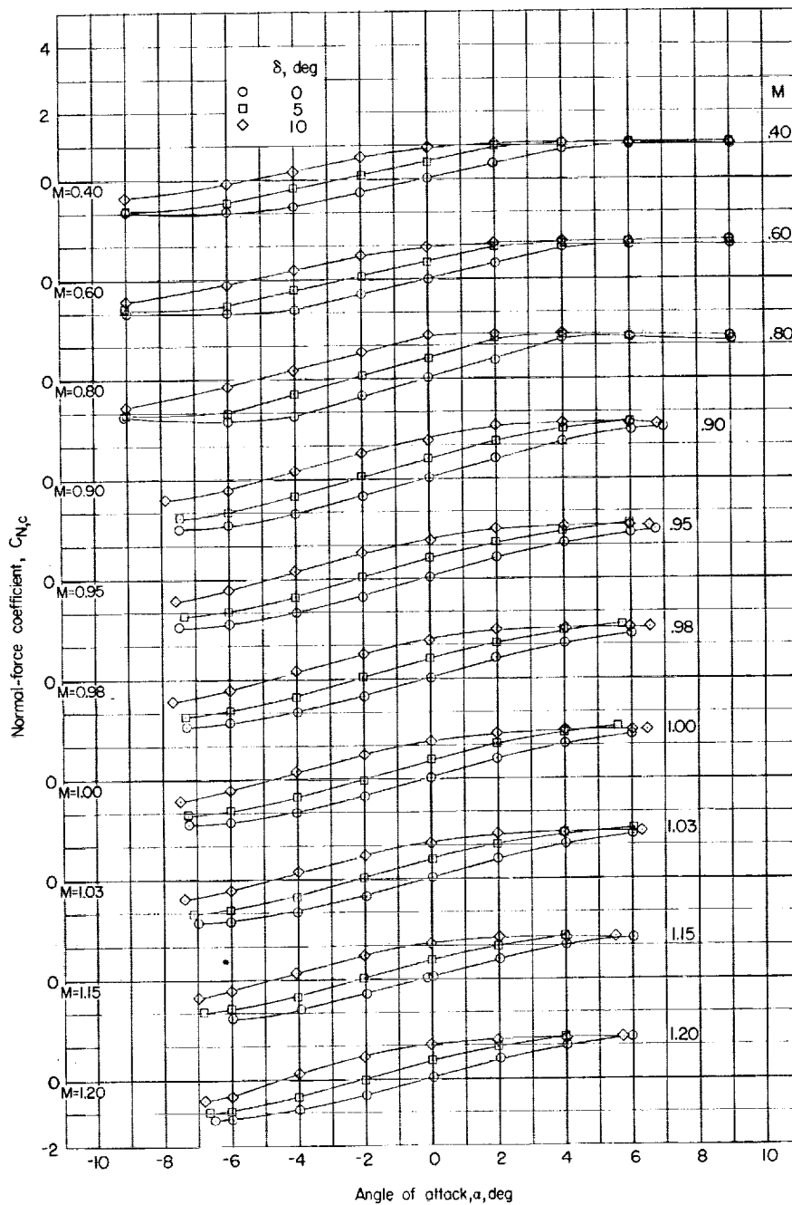
(d) Control surface 4.
