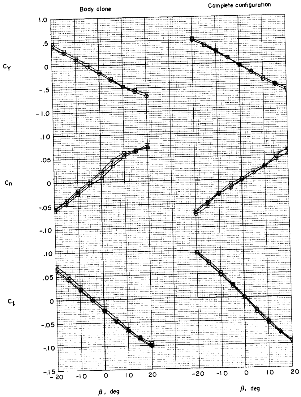
(d) \alpha = 70^\circ to \alpha = 90^\circ .
