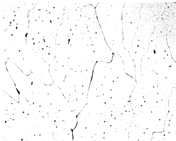
(e) Tungsten - 0.47 atomic percent boron. X100.
