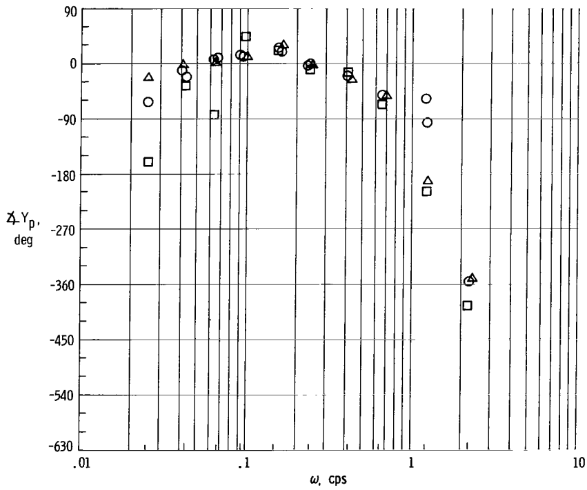
(d) Controlled element A-2* ground, run 60.
