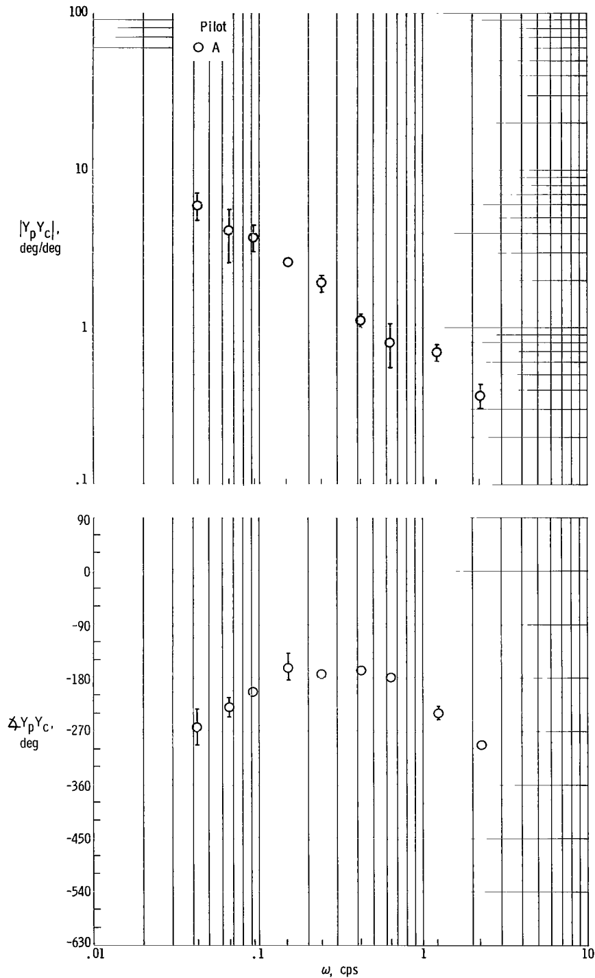
(d) Controlled element \frac{K}{s(s - \frac{1}{T})} , contact analog.
