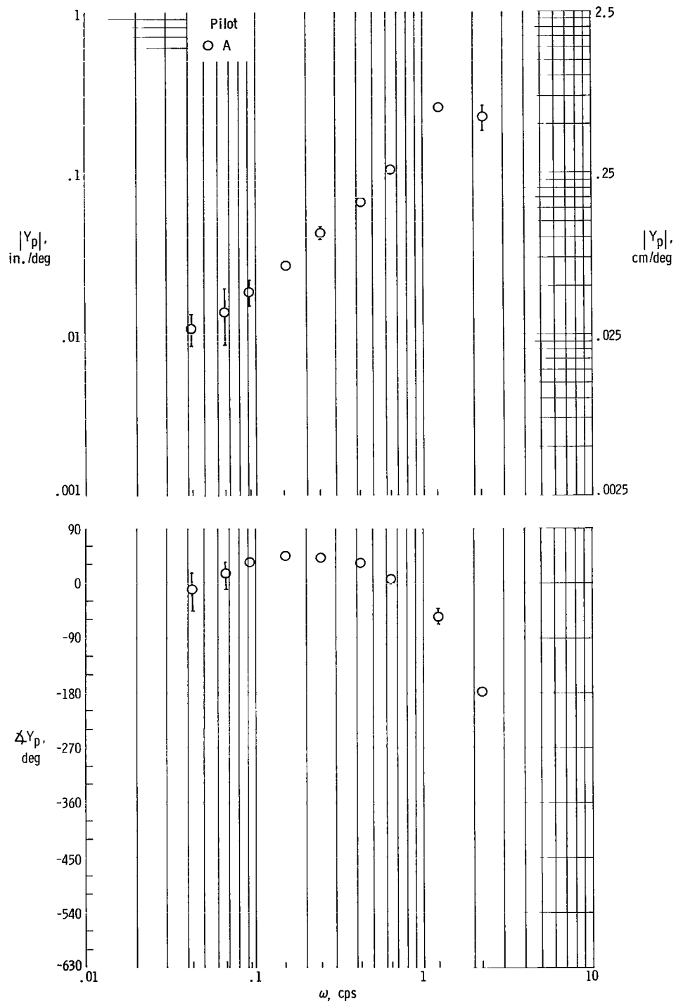
(d) Controlled element \frac{K}{s(s - \frac{1}{T})} , contact analog.
