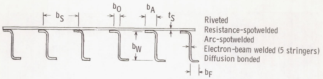
Z-stringer
