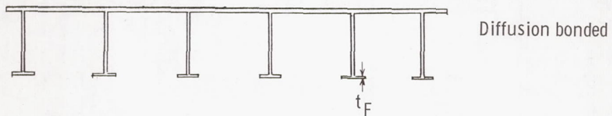
T-stringer
