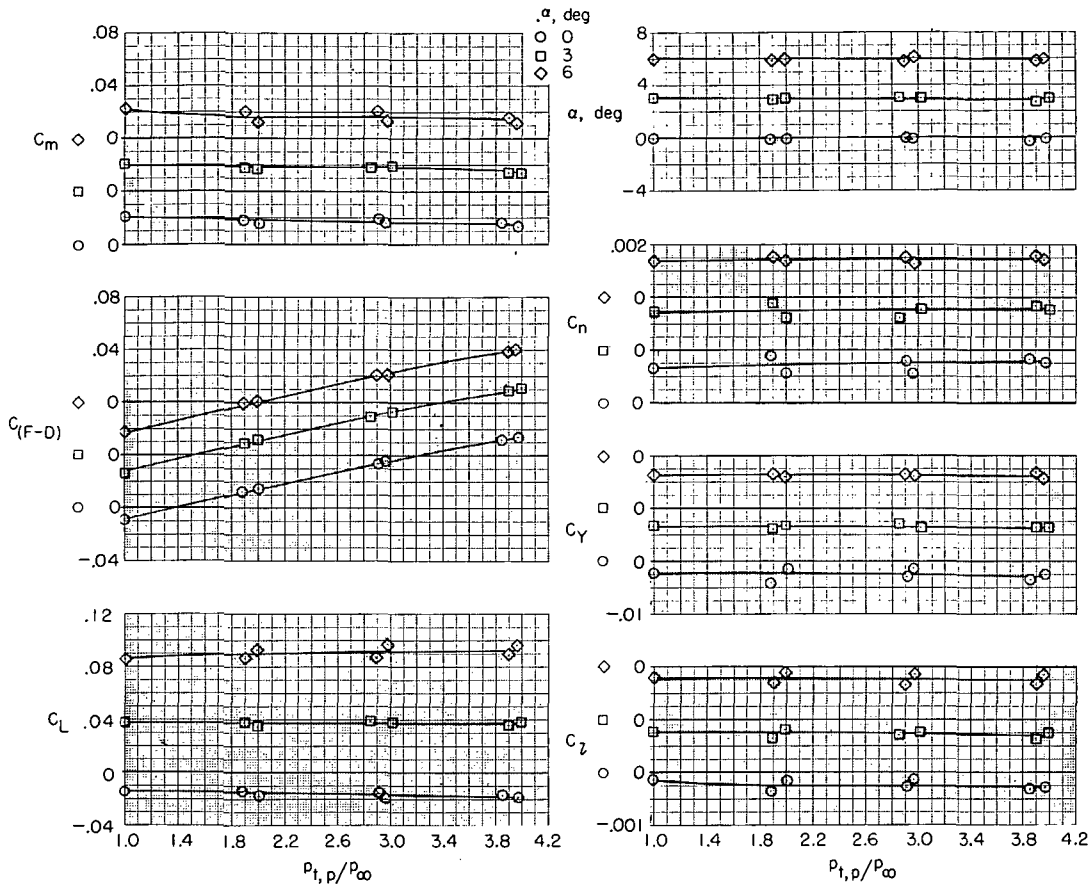
(d) M = 0.90 ; military power.
