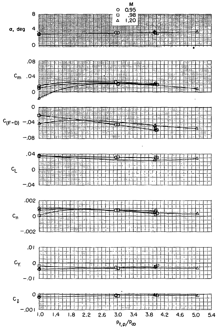
(d) M = 0.95 to 1.20 .
