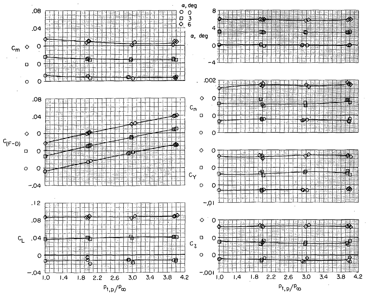
(d) M = 0.90 ; military power.
