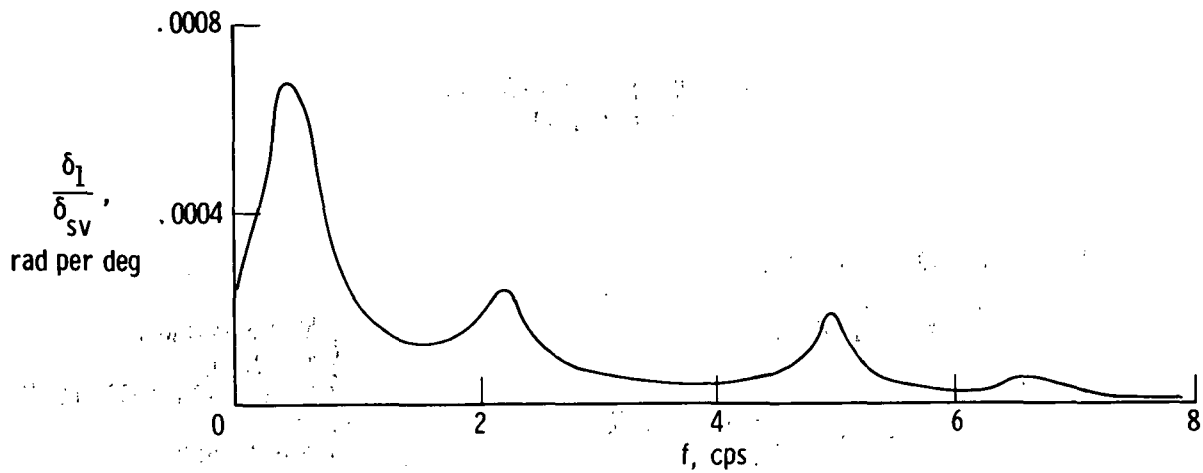
(a) Inboard elevon.
