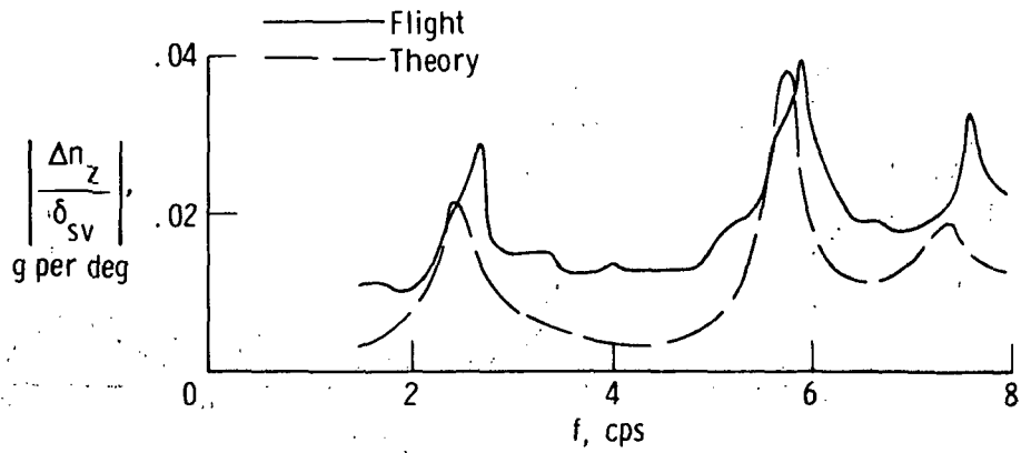
(d) Left wing; FS 56.18 m (2212 in.); BP 7.11 m (280 in.).
