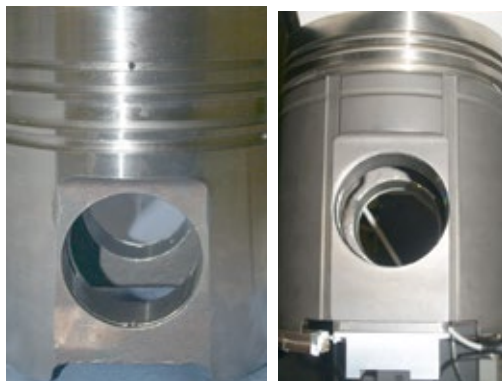
Abbildung 23: linke Seite: Kolben Variante 1 (Diesel- und Schwerölbetrieb), rechte Seite: Kolben Variante 2 (Gasbetrieb)
