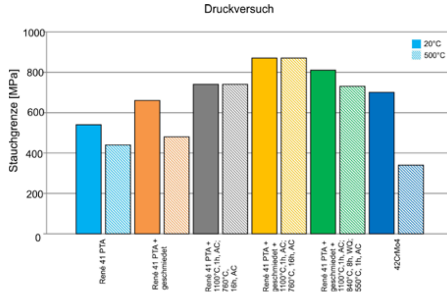
Abbildung 12: Einfluss einer Wärmebehandlung auf die Stauchgrenze Rp0,2
