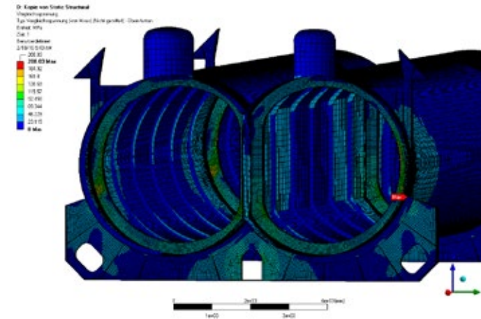
Abbildung 3: Strukturanalyse des Bilobe-Tanks mit FE-Methoden
