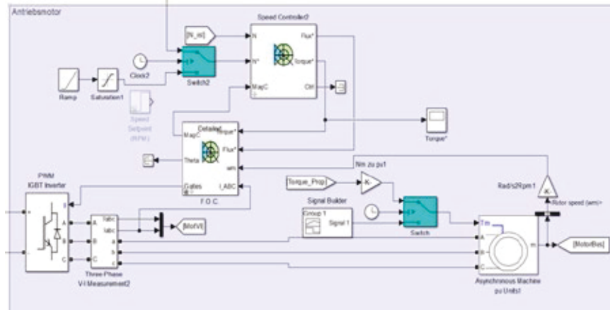
Abbildung 2: Modellbeispiel Antriebsmotor
