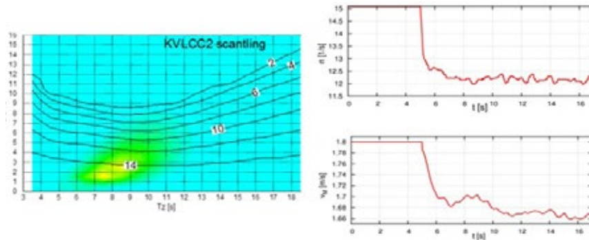
Abbildung 11: Erreichbare Geschwindigkeit eines VLCC Tankers abhängig von der signifikanten Wellenhöhe H_s und der mittleren Periode der Aufwärtswinddurchgänge T_z (links). Propellerdrehzahl (links oben) und Schiffsgeschwindigkeit (links unten) eines Kreuzfahrtschiffs bei unregelmäßigen Wellen von vorne (Ausschnitt aus einer Zeitreihe).
