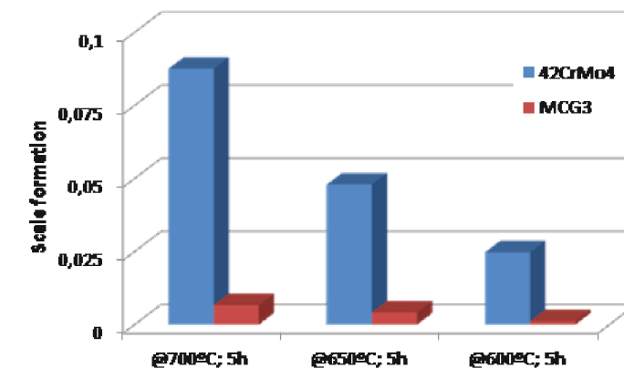
Abbildung 2: Vergleich der Oxidationsbeständigkeit von Proben 42CrMo4 und MCG3
