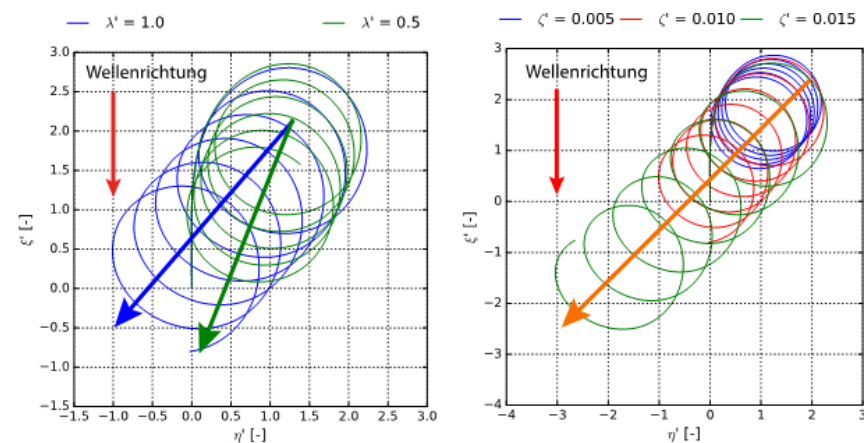
Abbildung 10: Simulierte Manöver in Wellen gleicher Steilheit (links) und gleicher Länge (rechts).
