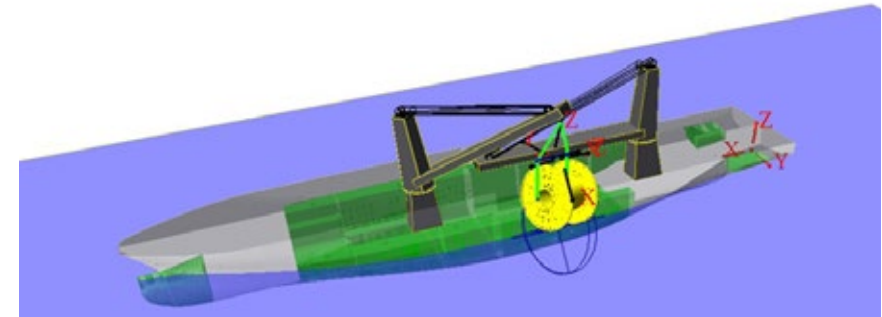
Abbildung 3 : Beispiel der Berechnung einer Umschlagsoperation mit einem Mehrkörpersystem (Traverse und Ladung) mit nicht korrekten Schwerpunktsannahmen.
