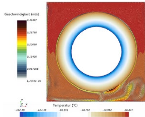
Abbildung 2: CFD-berechnetes Geschwindigkeitsfeld und Temperaturverteilung im Laderaum
