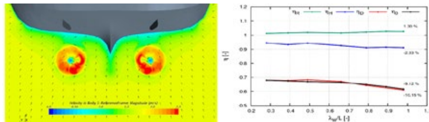
Abbildung 5: Kreuzfahrtschiff bei Fn=0,223 : Strömungsgeschwindigkeit kurz hinter der Propellerebene (links). Verlauf von \eta_D , \eta_R , \eta_H sowie \eta_0 in regelmäßigen Wellen (rechts).
