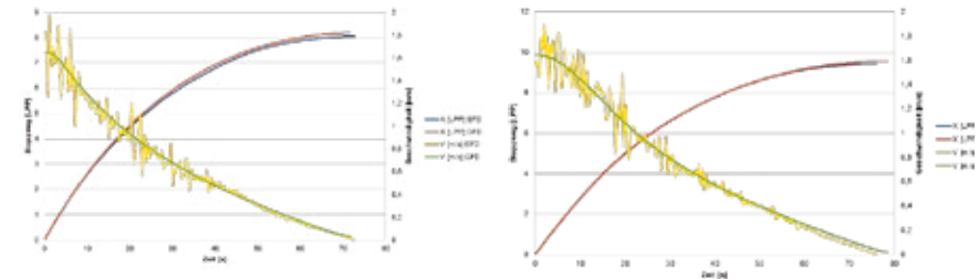
Abbildung 9: Vergleich von Geschwindigkeit und Stoppweg aus Simulation und Experiment, Verstellgeschwindigkeit 2°/s (links) und 8°/s (rechts)
