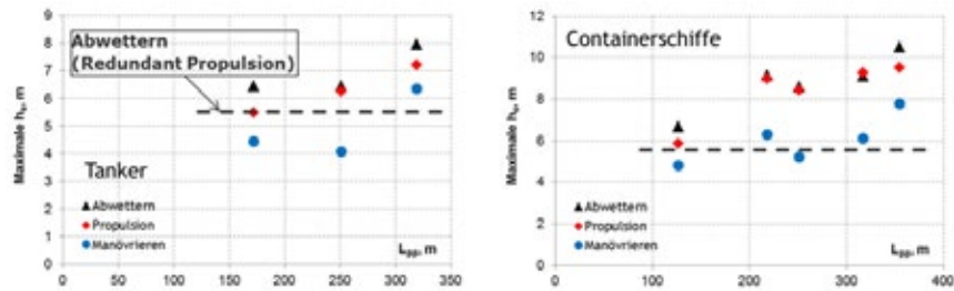
Abbildung 9. Erfüllung der Kriterien „Abwettern“, „Propulsion“ und „Manövrieren“ für Tanker (links) und Containerschiffe (rechts).
