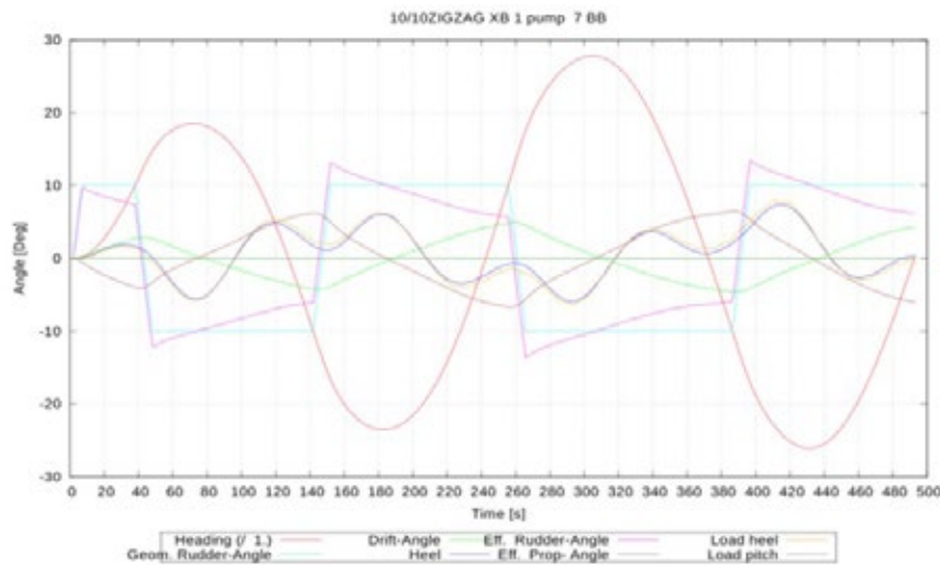
Abbildung 7 : Pendelnde Lastbewegung bei einem Zick-Zack-Manöver.
