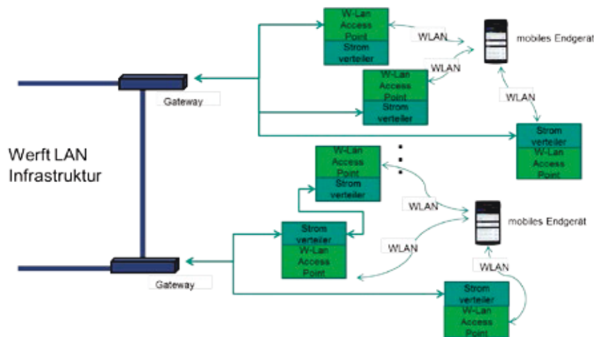
Abbildung 5: Konzept eines flächendeckenden Kommunikationssystems für die Anbindung an Bestandssysteme .
