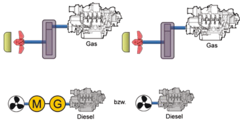
Abbildung 9: K13, Zweischauber mit Gasmotor; Diesel, bzw. Diesel-elektrisches Bugstrahlruder
