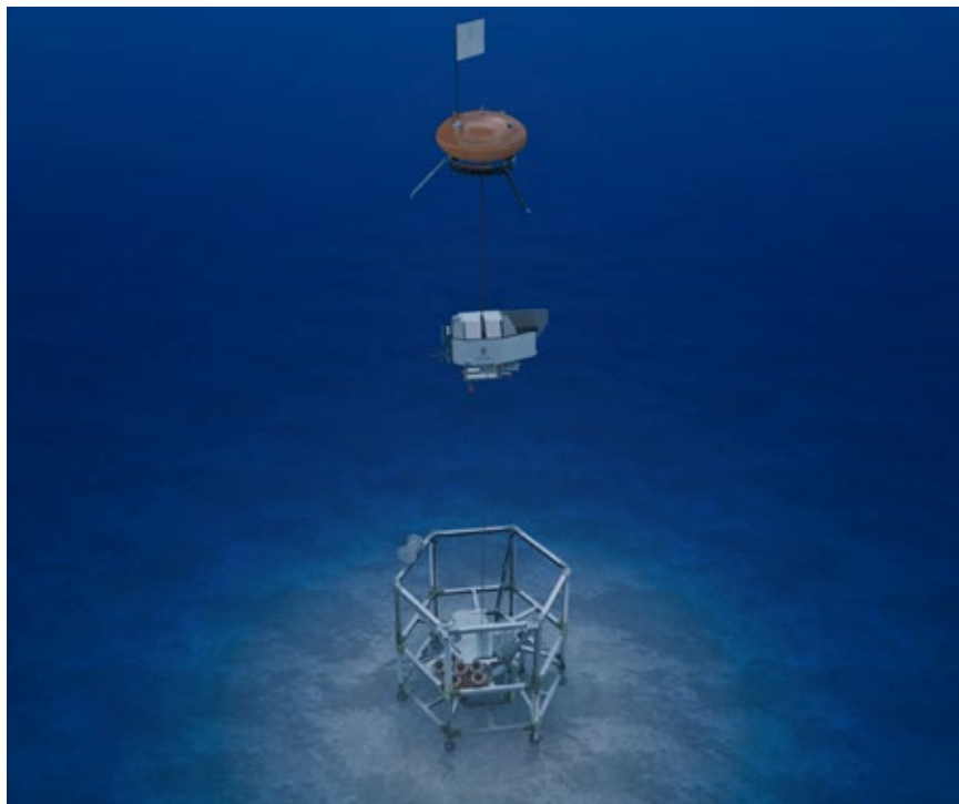
Abbildung 1: Rendering eines aktiven FlexMoT-Profiler-Systems.
