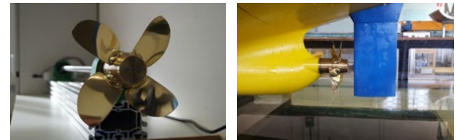
Abbildung 7: Entwickeltes dynamisches Verstellpropellersystem
