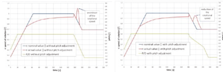
Abbildung 11: Steigungs- und Drehzahlverlauf im Stoppmanöver
