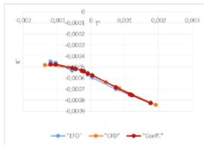
Abbildung 4: Längskraft X' am Schiff bei 10 kn und der Variation des Propellerschubzustands T'
