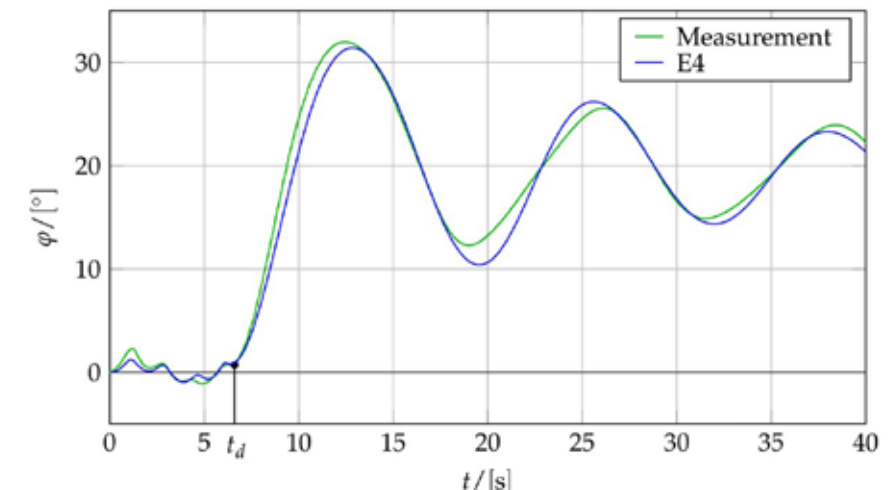
Abbildung 10 : Vergleich des gemessenen und berechneten Rollwinkels bei abreißender Kranlast.
