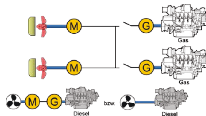
Abbildung 8: K15, Gas-elektrischer Hauptantrieb; Diesel, bzw. Dieselelektrisches Bugstrahlruder
