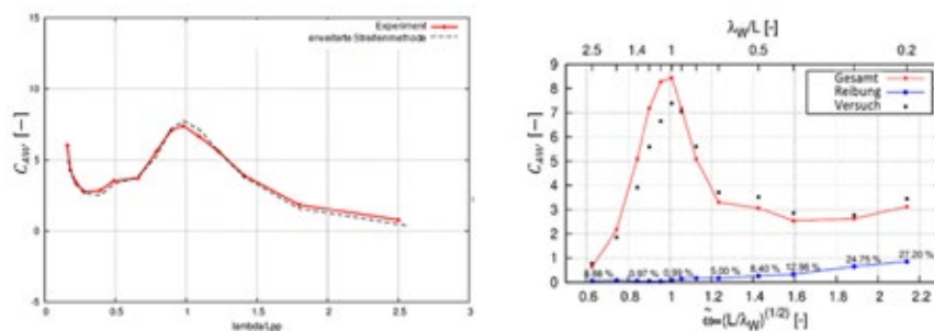
Abbildung 3: Quadratische Übertragungsfunktion des wellenbedingten Zusatzwiderstands in Wellen von vorne, Streifenmethode (links) und RANSE-Verfahren (rechts).
