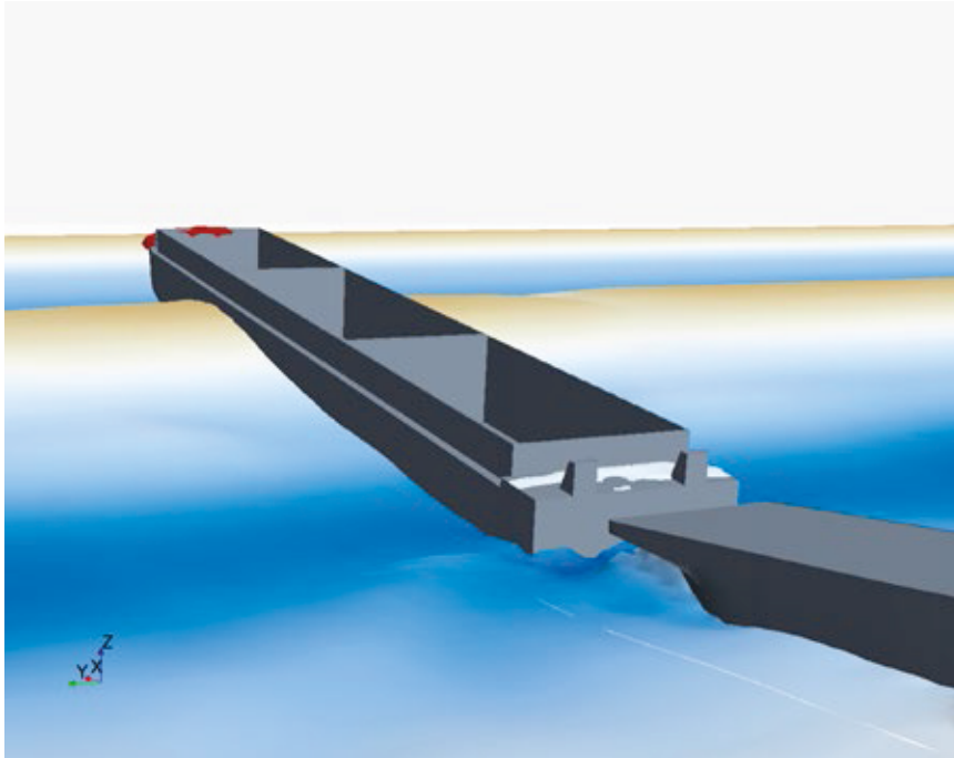
Abbildung 6: Exemplarische Visualisierung aus einer numerischen Simulation für den gelenkig gekoppelten Verband im Seegang.
