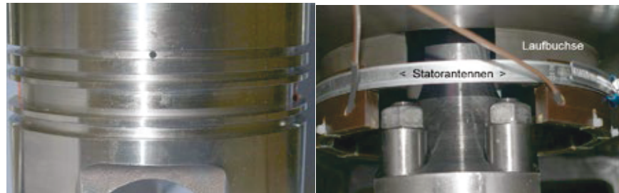
Abbildung 6: Kolben aus MCG3 im Prüfmotor im WTZ
