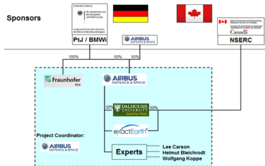
Abbildung 4: Projektstruktur
