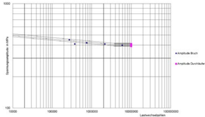
Abbildung 20: Wöhlerkurve für den Werkstoff MCG3 für eine Zug-Druck-Wechselfestigkeitsbeanspruchung
