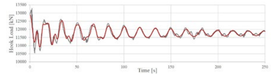
Abbildung 9 : Vergleich von gemessenen und berechneten Hakenlast aus einem Rollauschwingversuch
