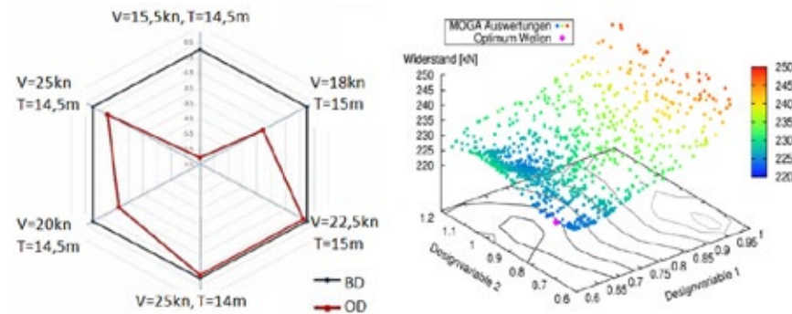
Abbildung 8: Veränderung des Gesamtwiderstands eines 14.000 TEU Containerschiffs bei verschiedenen Betriebsszenarien (links). Gesamtwiderstand eines Offshore-Versorgers abhängig von zwei Designvariablen (rechts).
