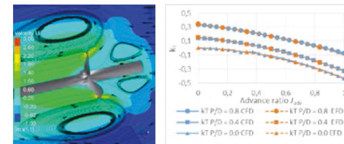
Abbildung 6: Strömungsfeld um Propeller (links), Freifahrtkurven (rechts)
