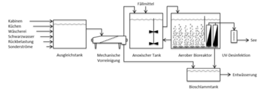
Abbildung 1: Konfiguration einer modernen Schiffskläranlage (Köster et al., 2016)
