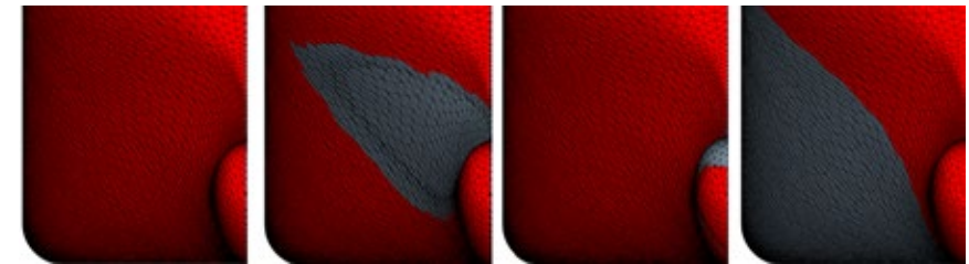
Abbildung 7: Beispielhafte Veränderung der Buggeometrie eines 14.000TEU Containerschiffs.
