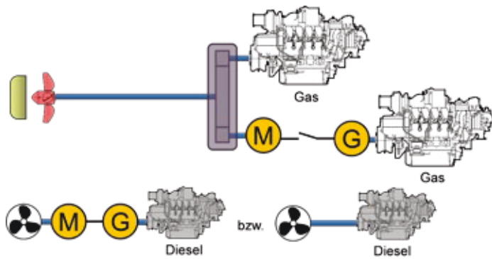
Abbildung 10: K5, Gasmotor als Hauptantrieb mit Power-Take-In Gasmotor; Diesel, bzw. Diesel-elektrisches Bugstrahlruder
