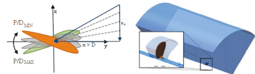
Abbildung 5: Änderung Propellersteigung (links), Rechendomain (rechts)
