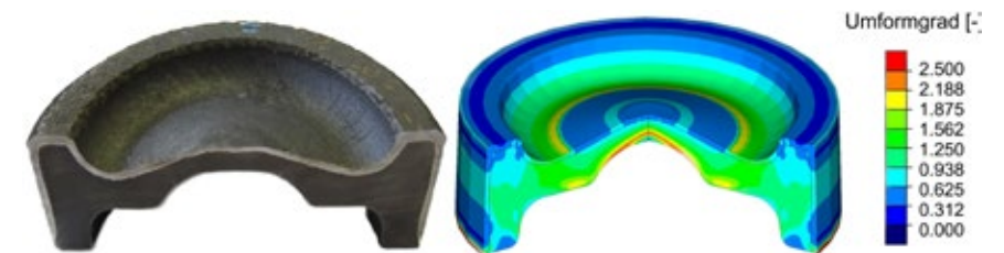
Abbildung 14: Vergleich Realbauteil mit Simulationsmodell
