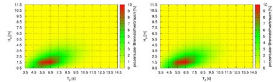
Abbildung 1: Prozentualer Brennstoffverbrauch auf der Route „World-Wide Trade“ für ein 14.000 TEU Containerschiff (links) und ein 707 TEU Containerschiff (rechts).
