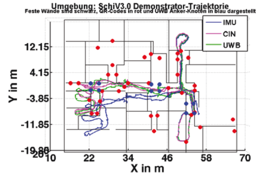
Abbildung 4: Trajektorie aufgenommen während der Demonstrator-Evaluation. Die schwarzen Linien stellen dabei den Grundriss dar. Die Kurve in Blau wurde durch IMU-Daten gewonnen, die rosa Kurve stellt die stabilisierte passive Lokalisierung mit Check-Ins an QR-Codes (rote Punkte) und die grüne Kurve die aktive Lokalisierung mit UWB Knoten (blaue Punkte) dar.
