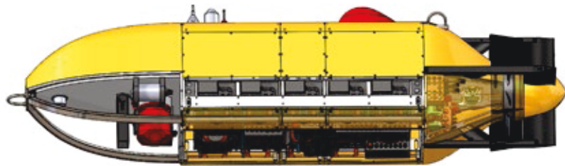
Abbildung 4: AUV 'Doris alpha' mit geöffneten Kompartments für Nutzlast, Batterie und Antriebssystem (Quelle: Enitech)
