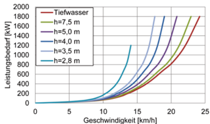
Abbildung 5: Exemplarische Kurvenschar aus der Modellierung für das 135 m Schiff bei 2 m Tiefgang.
