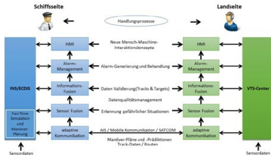
Abbildung 3: COSINUS-Systemarchitektur
