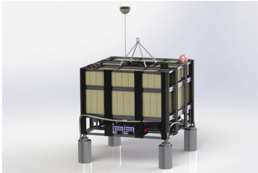
Abbildung 6: Basismodul der SBS mit vier Sauganker-Füßen (3D CAD Modell) (Quelle: TU Berlin).
