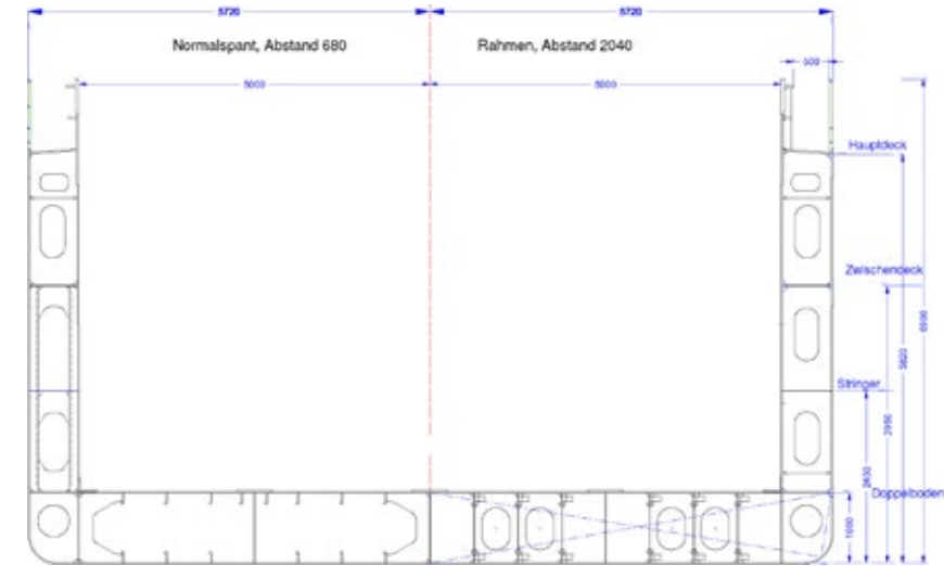
Abbildung 4: Hauptspantkonstruktion der finalen Version HH.
