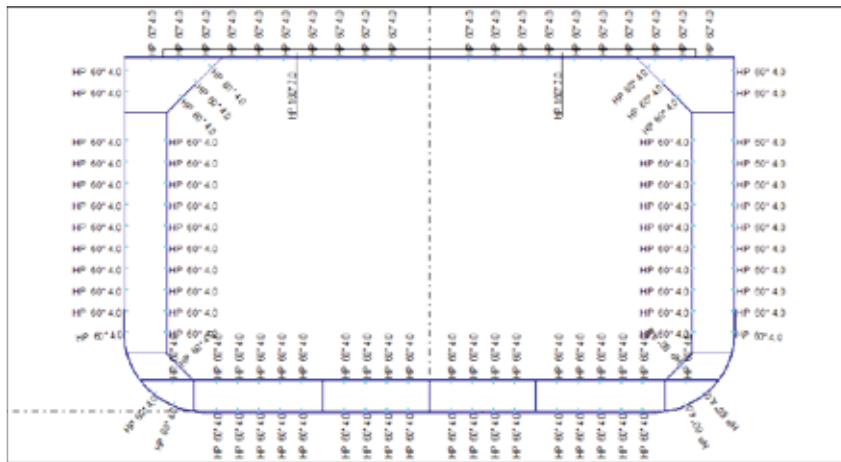
Abbildung 12: Steifen im Bereich des Hauptspantes
