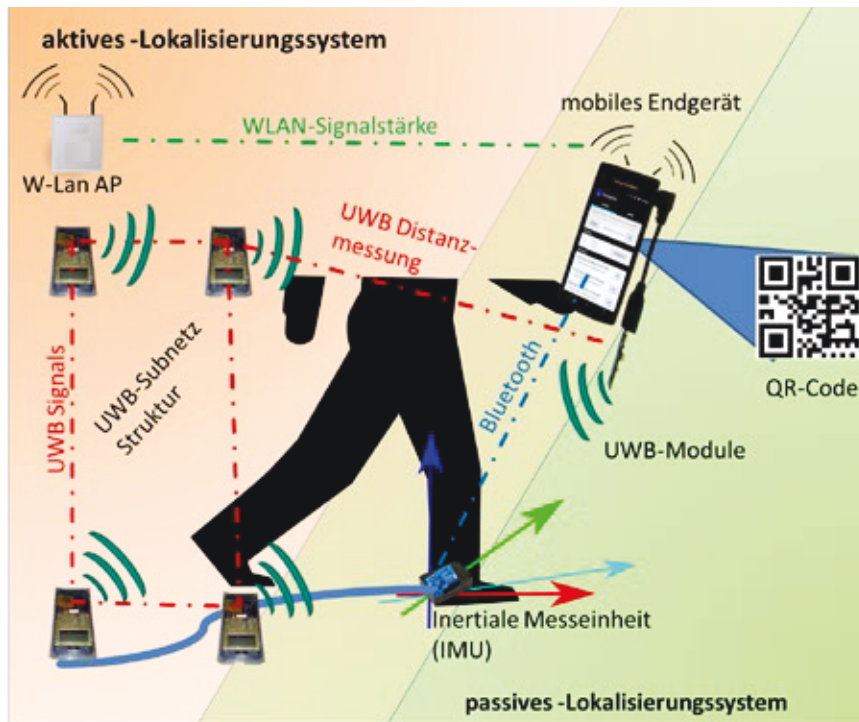
Abbildung 3 Aktives und passives Lokalisierungssystem als unterschiedliche Ausbaustufen eines hybriden Lokalisierungssystems
