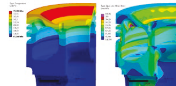
Abbildung 17: Ergebnisse aus Extremlastfall Temperaturfeld + Gaskräfte, links: Temperaturfeld °C, rechts: von Mises Spannung N/mm 2
