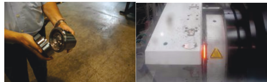
Abbildung 5: Reibschweißteile, Oberteil MCG3 und Unterteil MCG3 Reib- schweißung auf Schwungradreibschweißmaschine bei GSA
