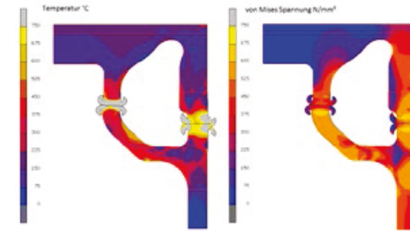
Abbildung 16: Ergebnisse, links: Temperaturfeld nach Reibschweißprozess (Temperatur °C), rechts: Eigenspannungen in kaltem Zustand (von Mises Spannung N/mm 2 )
