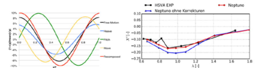
Abbildung 4: Überlagerung der Nachstromanteile über eine Periode (links). Vergleich der mittleren Längskraft mit Messungen der HSVA ( \alpha=30^\circ ), rechts.
