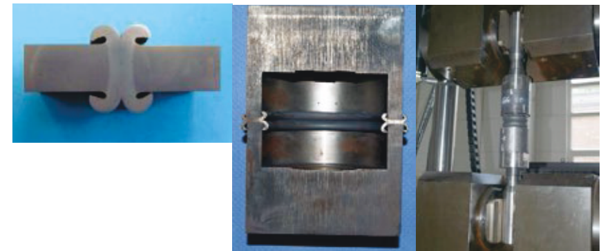
Abbildung 4 : Reibschweißverbindung MCG3 mit MCG3 mit Demonstrator- teil
