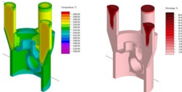
Abbildung 18: Ergebnisse der Gusssimulation für das Kolbenunterteil, links: Temperaturfeld °C nach 30s, rechts: Porositätsrisikozonen
