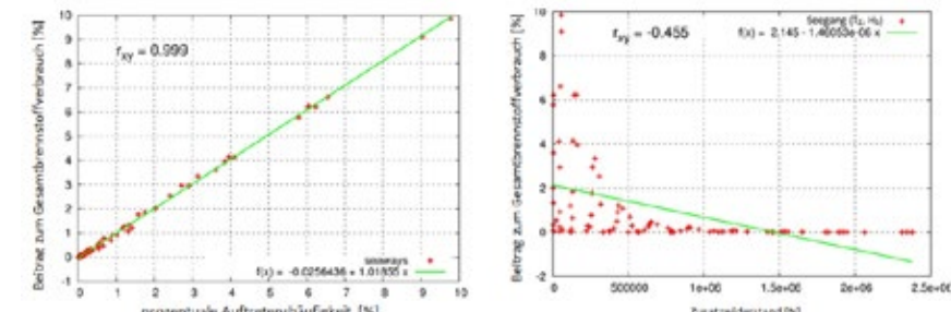
Abbildung 2: Lineare Korrelationen zwischen dem Beitrag zum Gesamtbrennstoffverbrauch (Ordinate) und der Auftretenshäufigkeit (links) sowie des seegangsbedingten Zusatzwiderstands (rechts).
