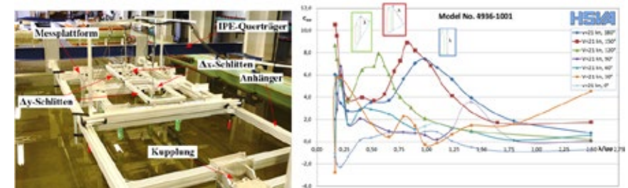
Abbildung 6: Messplattform der TUB (links). Übertragungsfunktion des Zusatzwiderstands in Wellen aufgetragen über dem Verhältnis Wellenlänge/Schiffslänge (rechts).
