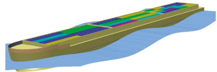
Abbildung 3: 3D-Ansicht des Leichters in Version E mit geteilten Laderäumen.
