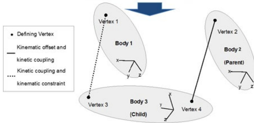
Abbildung 2: Prinzip des Mehrkörpersystems für das universelle Kranmodell
