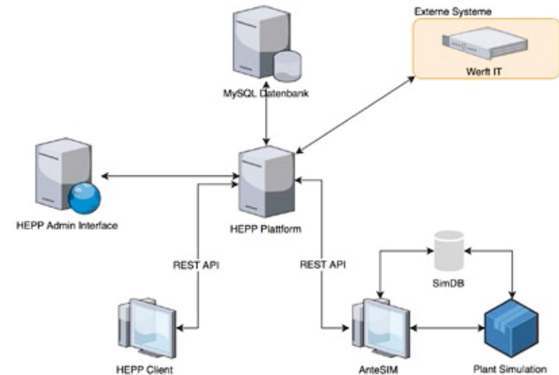
Abbildung 3: Übersicht HEPP-Plattform
