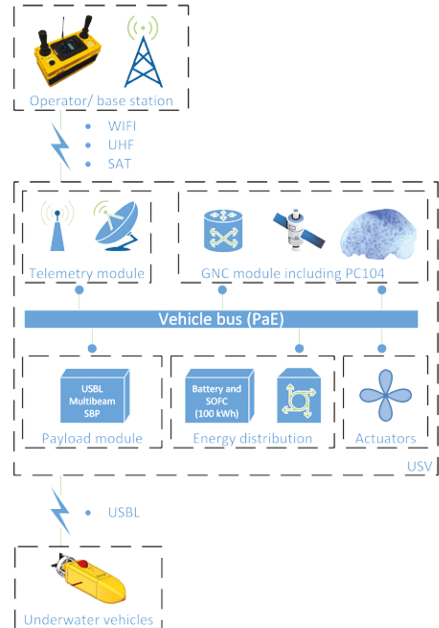
Abbildung 2: Automatisierungs- und Telemetrie-Konzept des USV (Quelle: Universität Rostock)
