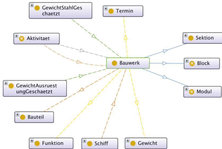
Abbildung 2: Ausschnitt aus der HEPP-Ontologie
