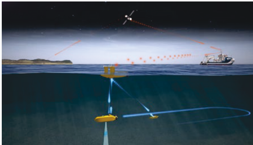
Abbildung 8: Illustration der verschiedenen Kommunikationswege innerhalb einer Mission (Quelle: IMPaC)
