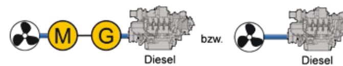
Abbildung 6: K1, Dieselmotor als Hauptantrieb; Diesel, bzw. Diesel-elektrisches Bugstrahlruder
