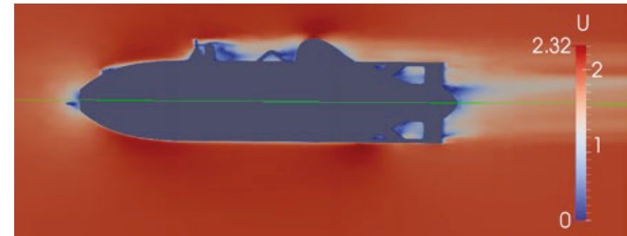
Abbildung 3: CFD-Analyse der Umströmung der AUVs 'Doris alpha und beta' (Widerstandskoeffizienten, Druck-, und Geschwindigkeitsverläufe) (Quelle: Enitech)
