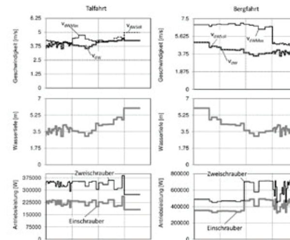
Abbildung 11: Zeitabhängige Geschwindigkeits- und Lastprofile für die Tal- und Bergfahrt
