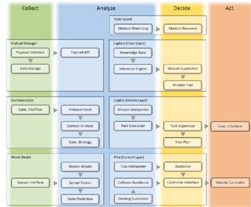
Abbildung 9: Modulare High-Level-Steuerungs-Architektur der SMIS-Fahrzeuge, gruppiert nach der üblichen Autonomie-Schleife Sense-Plan-Act (Quelle: KIT)
