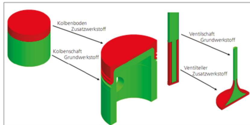
Abbildung 1: Werkstoffverbund - Demonstratorbauteile
