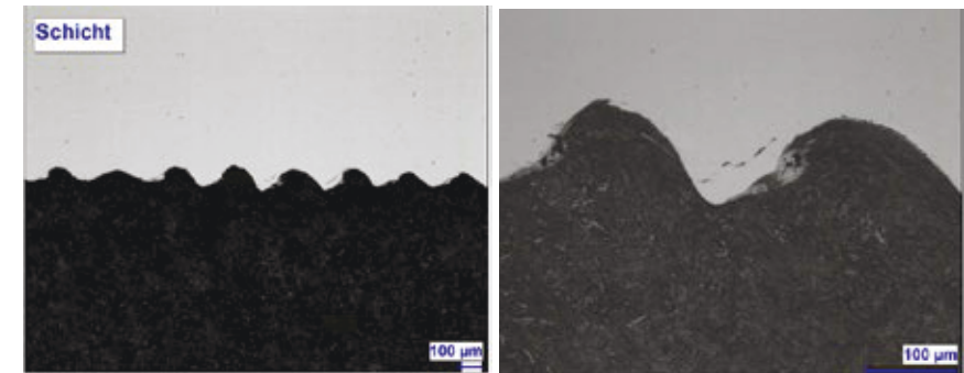
Abbildung 7: Turbulente Ausbildung der Bindezone einer Explosionsplattierung
