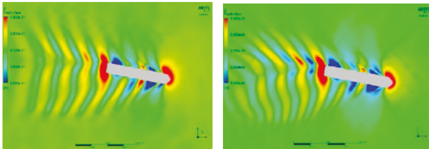
Abbildung 3: Schiffswellensystem bei 14 kn bei Drift (links) und kombinierter Drift- und Gierbewegung (rechts) im Modellmaßstab
