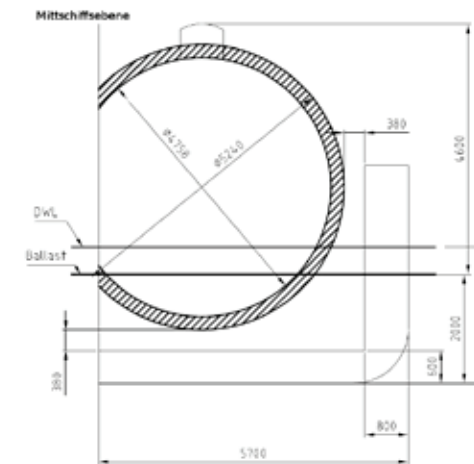
Abbildung 1: Bilobe-Tank im Querschnitt
