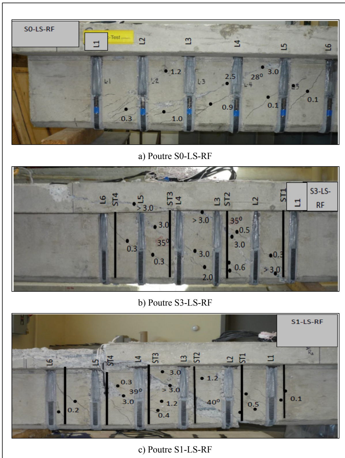
Figure 5. 4 Fissuration mesurée dans les poutres LS-RF
