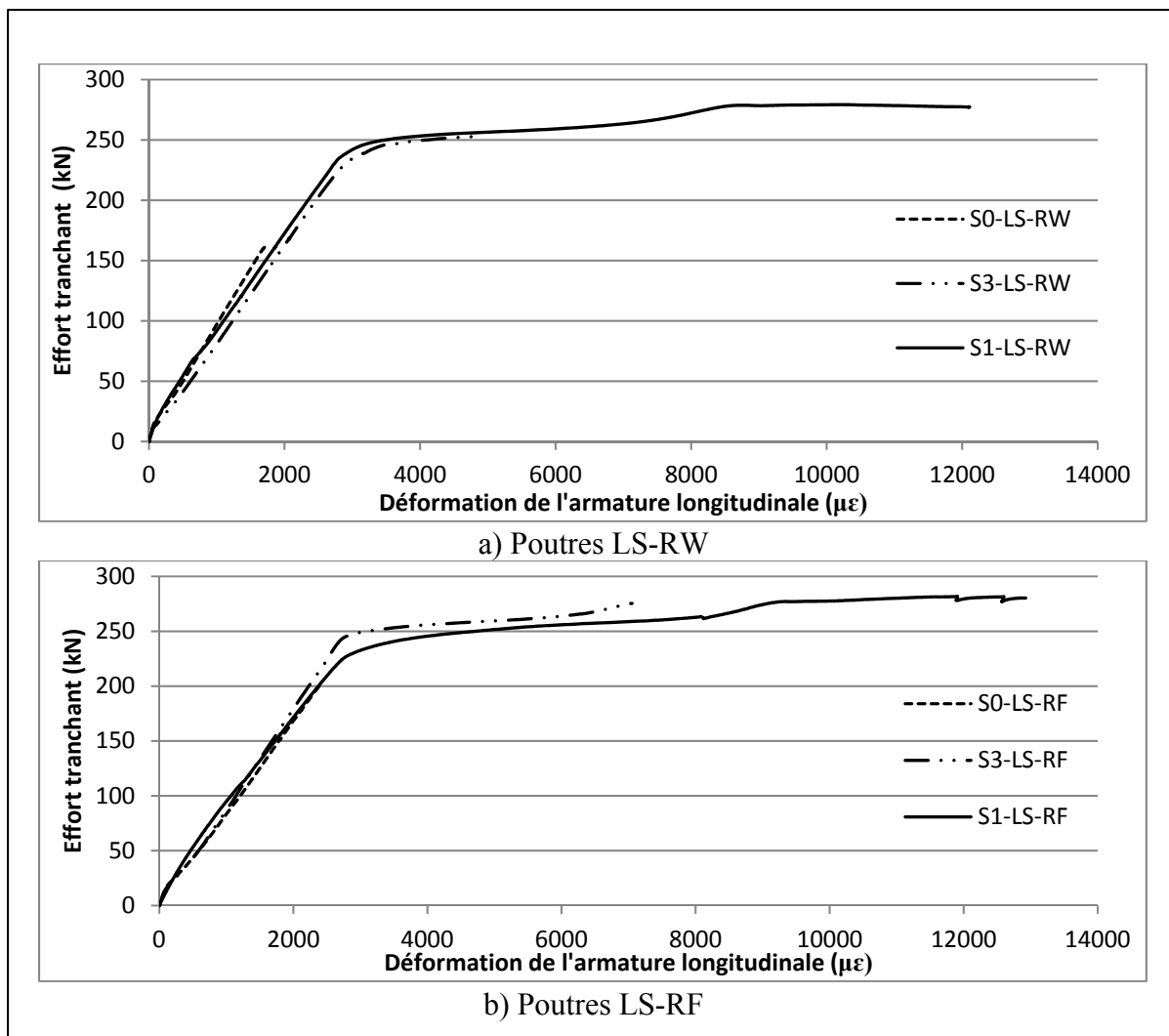
Figure 4. 2 Déformation de l'armature longitudinale au droit de la charge
