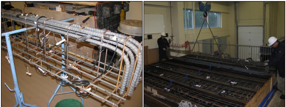
Figure 3. 3 Montage de l'armature et du coffrage
