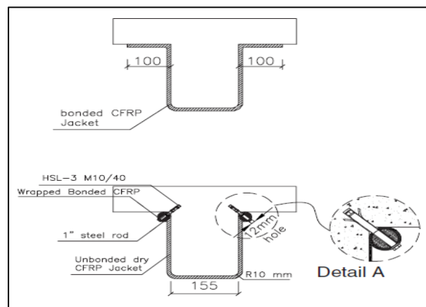
Figure 2. 3 Systèmes de renforcement proposé Tirée de Galal et Mofidi (2010)
