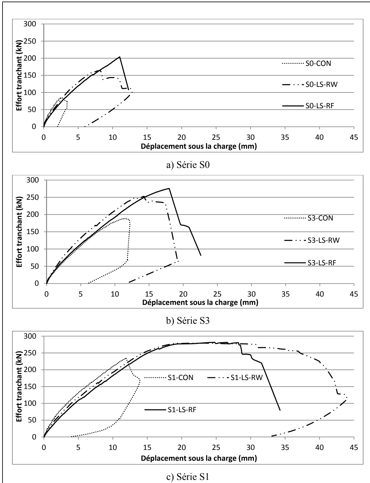
Figure 4. 1 Courbes effort-déplacement sous la charge
