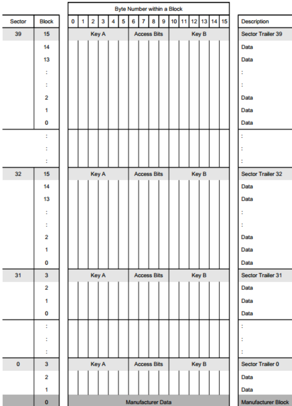
Figure 15 : Structure de la mémoire d'un badge MIFARE 4K
