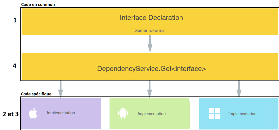
Figure 24 : Implémentation du service de dépendance
