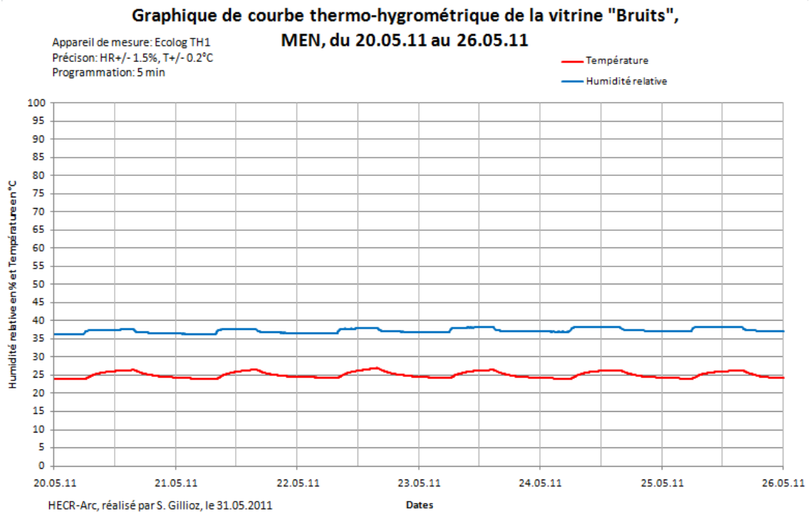
III. 18 Graphique de courbe thermo-hygrométrique de la vitrine « Bruits » (©HECR Gillioz, 2011)
