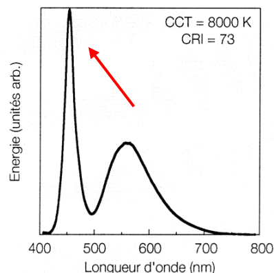
Ill. 6 Spectre d'émission d'une source LED blanche à très haute efficacité, (©Ferrini, 2010, p.38.)
