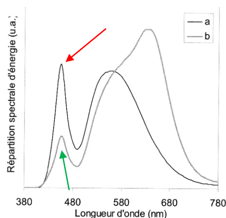
III. 7 Répartition spectrale d'énergie relative de deux sources LED blanches : a) LED blanc froid à un phosphore, Tc environ 5'500 K, b) LED blanc chaud à plusieurs phosphores, Tc environ 2'750 K, (©Viénot, 2008, p.220.)
