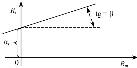
Рис. 3. Характеристична лінія для визначення \beta -коефіцієнта
