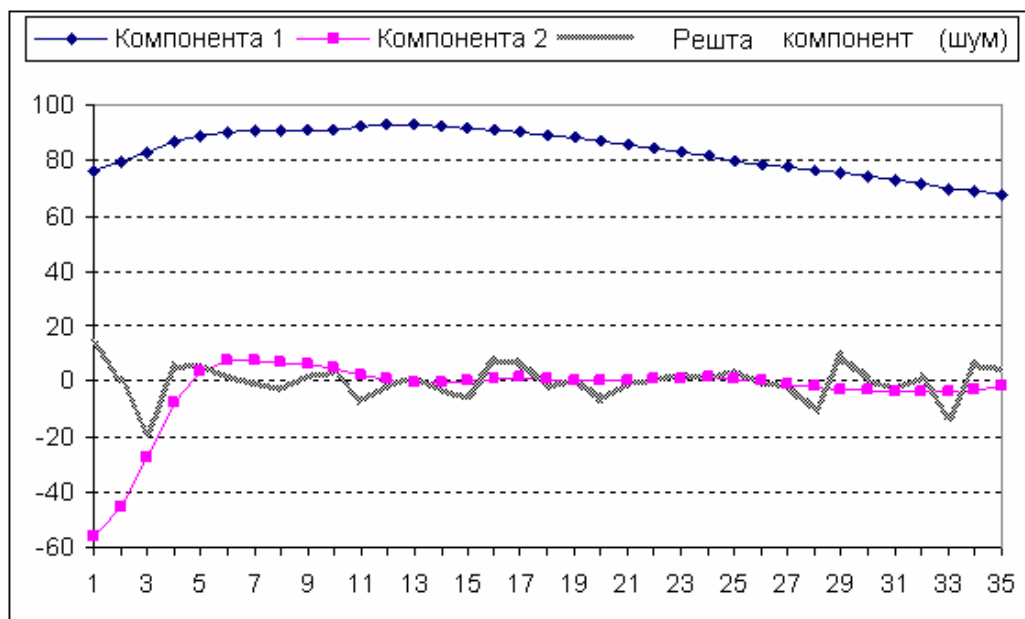
Рисунок 2.3 – Компоненти ряду
