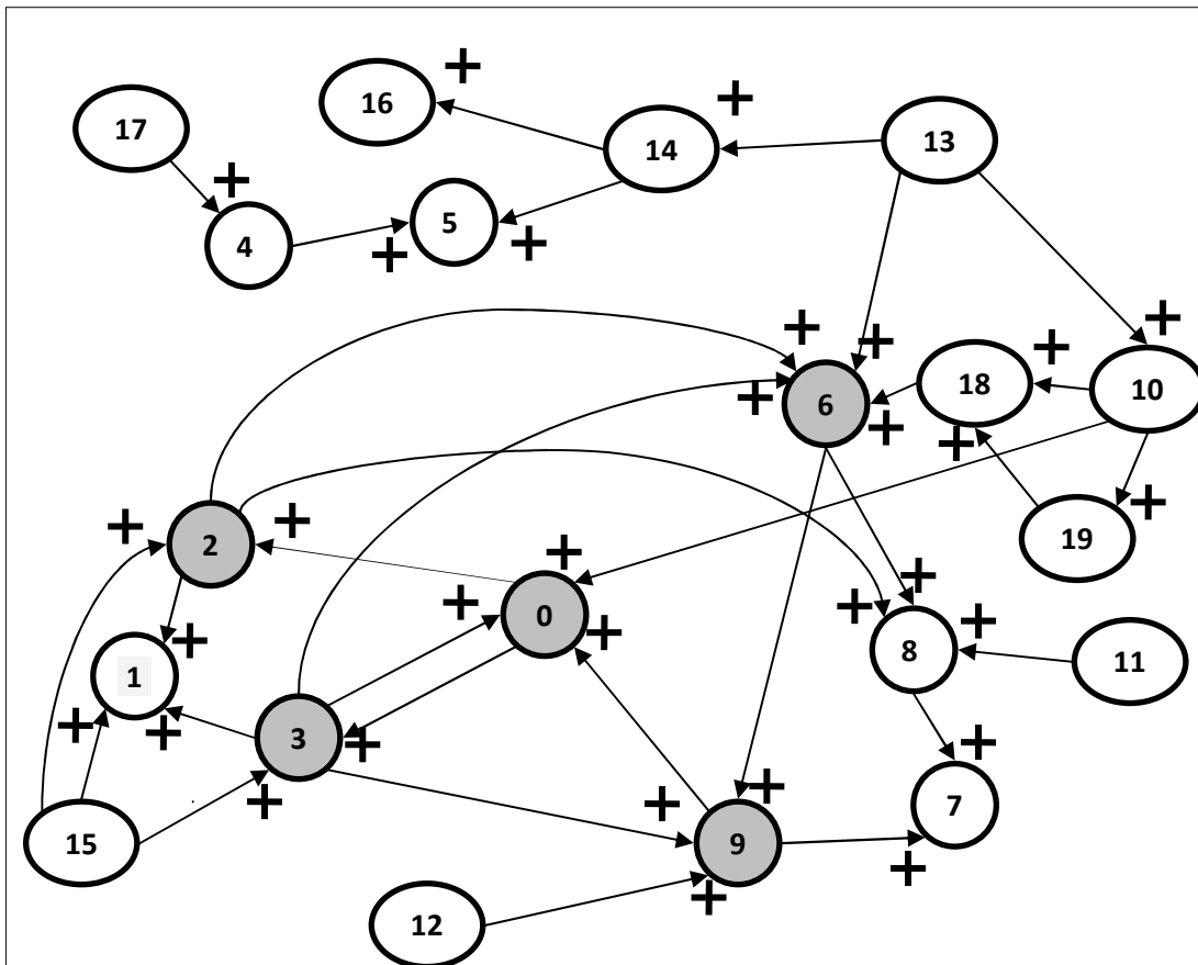
Рисунок 3.3 — Знаковий граф
