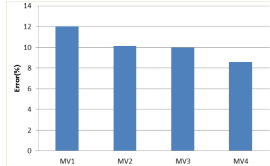
Fig. 33 PN model prediction error
