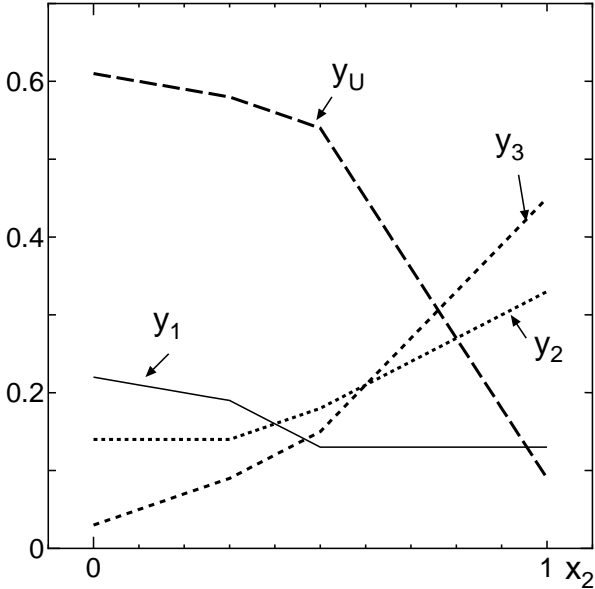
図 2 数値例 2 y_j = f_{\mu_j^{\circ}}^{EC}(0.5, x_2, 0.3) のグラフ
