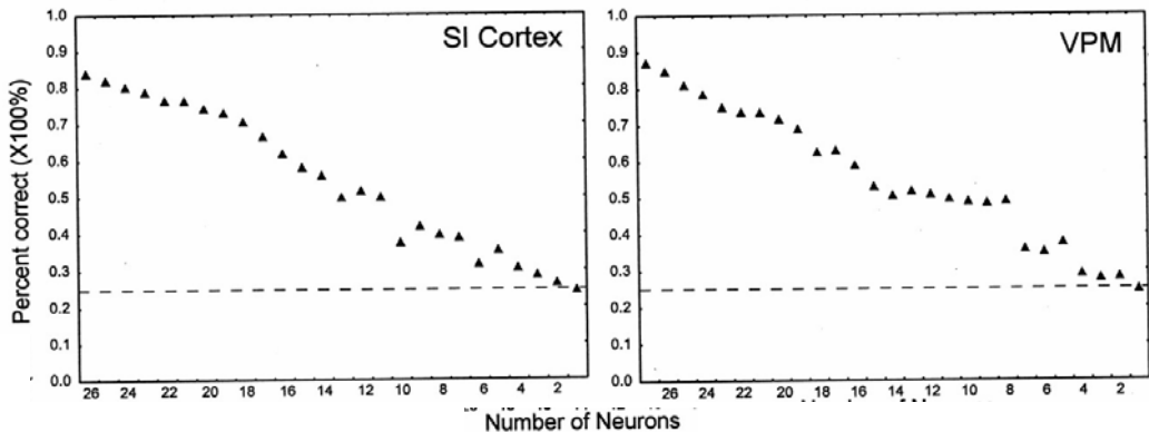
图 3 皮层和丘脑神经元群对胡须触觉的辨别能力
