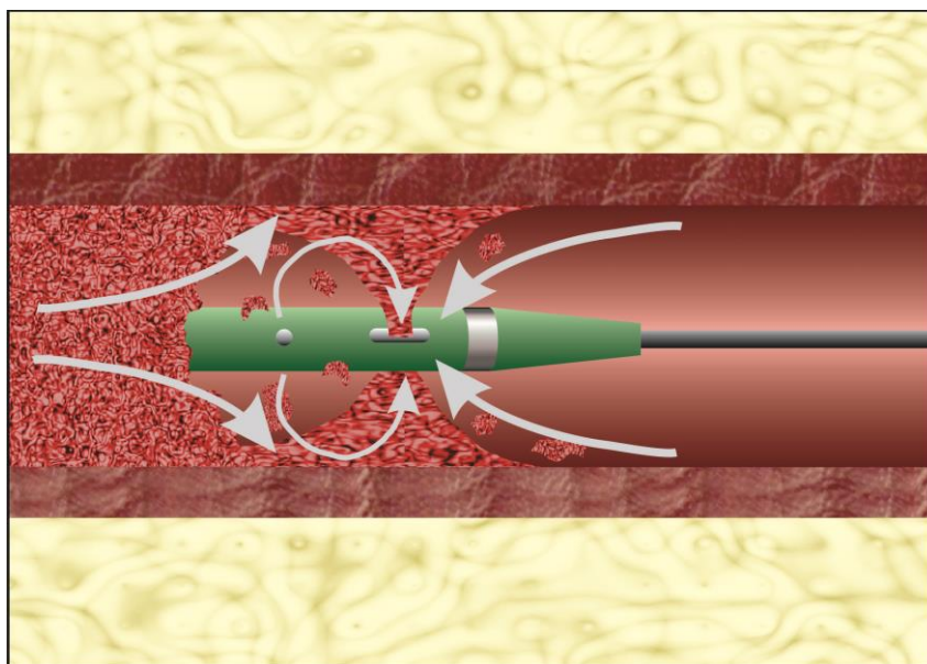
Figura 3 - Esquema de funcionamento por aspiração de Venturi dos cateteres tipo AngioJet ® e o Hidrolyser ® . Desenho, Luiz F. Farret.
