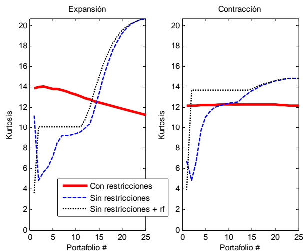
Kurtosis de los retornos diarios de los portafolios de las fronteras eficientes
