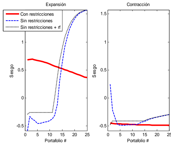
Sesgo de los retornos diarios de los portafolios de las fronteras eficientes
