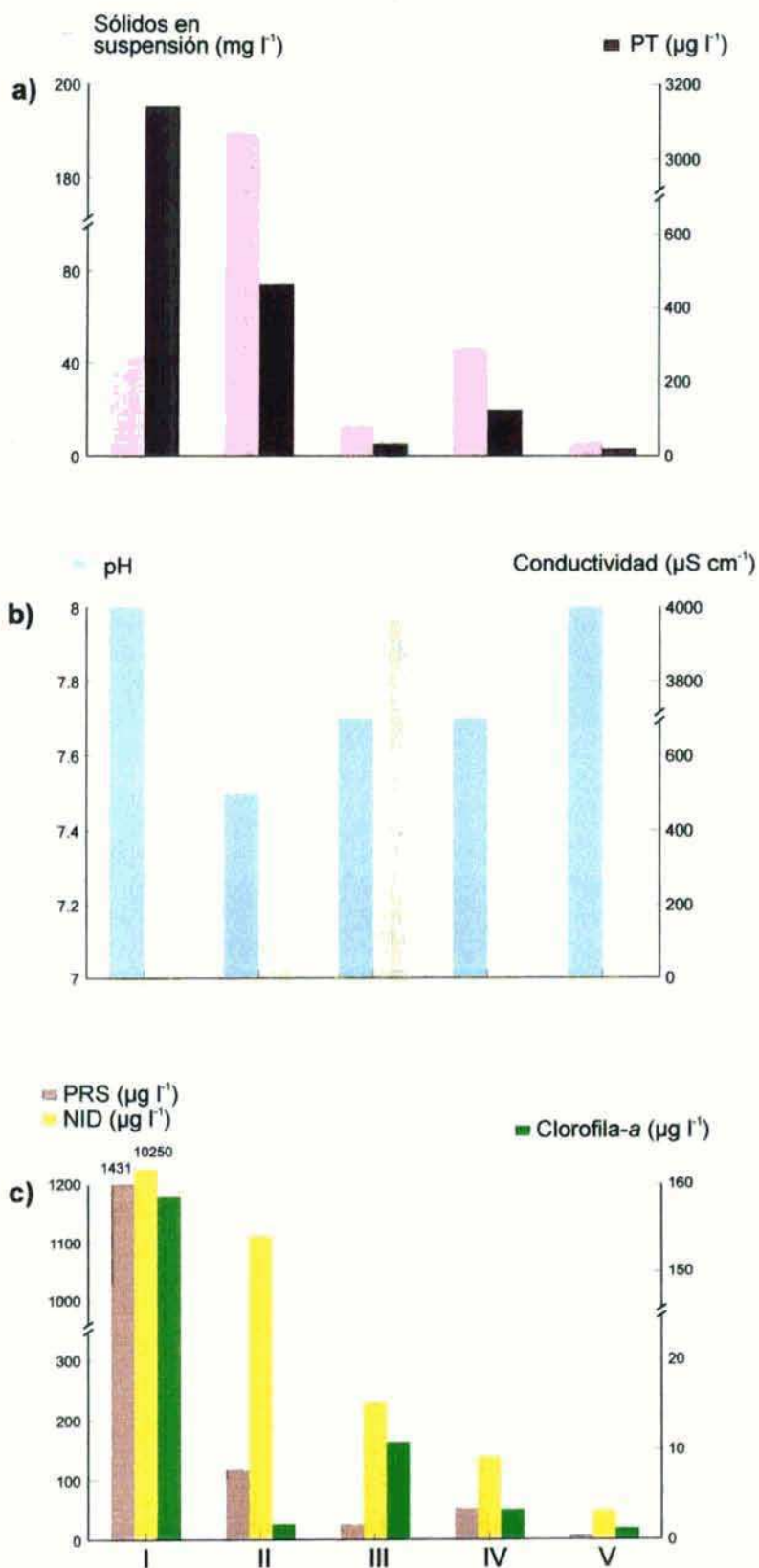
Fig. 21 : a- Sólidos en suspensión y fósforo total; b- pH y conductividad; c- Fósforo reactivo soluble, nitrógeno inorgánico disuelto y clorofila-a para cada grupo de lagos resultante de la ordenación a partir del PCA.
