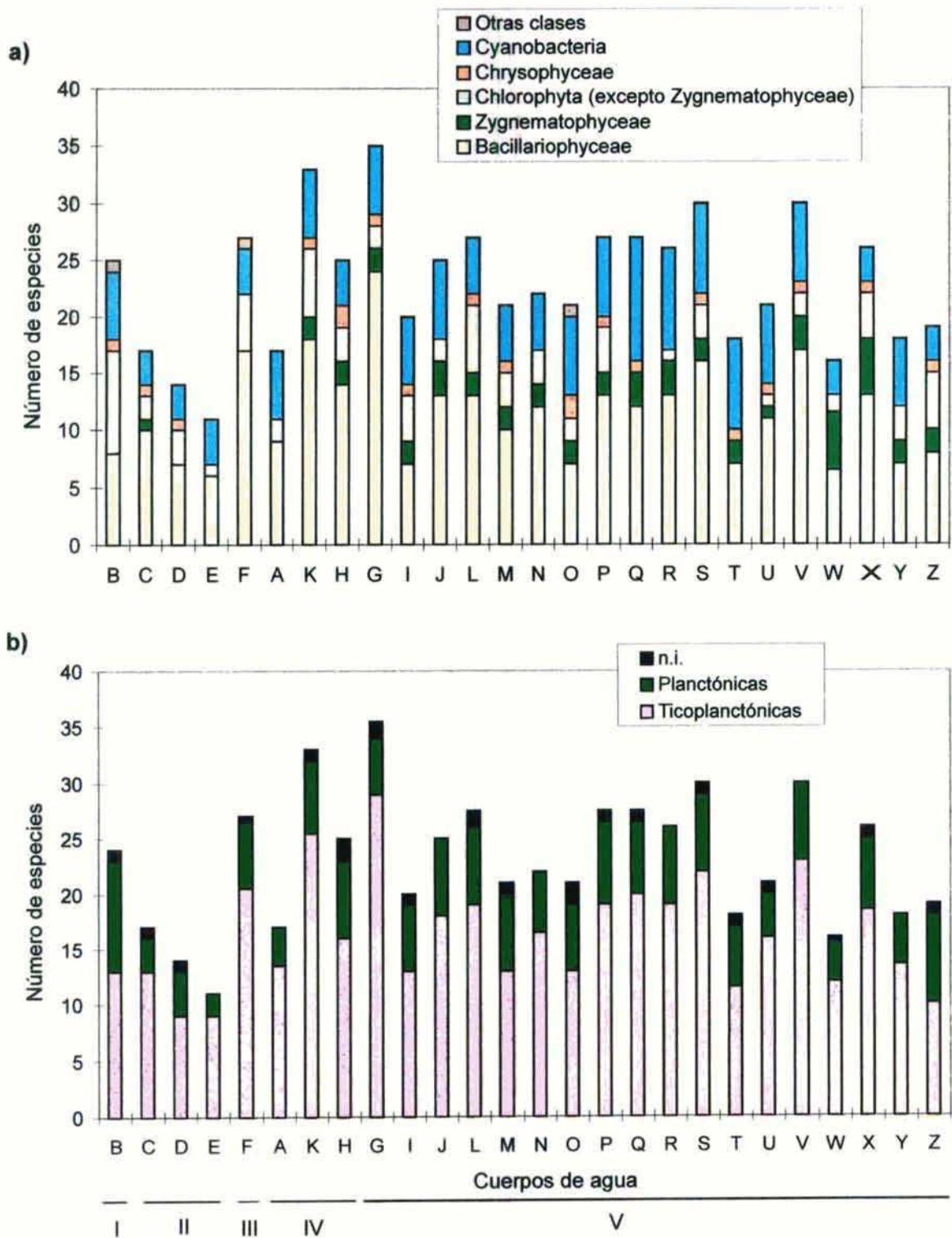
Fig. 18 : a- Riqueza específica por grupo algal; b- Número de especies planctónicas, ticoplanctónicas y no identificadas (n.i.). Grupos I-V: grupos de cuerpos de agua obtenidos a partir del PCA.
