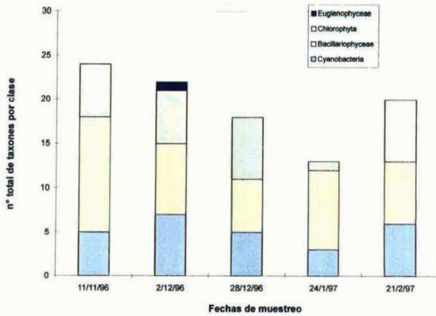
Fig. 43 : Variación temporal del número total de taxones por grupo algal en la Laguna B.
