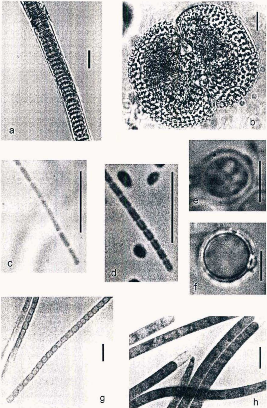
Fig. 17 : a- Prasiola crisper (Lightf.) Menegh.; b- Cosmarium dentiferum Corda; c- Leptolyngbya angustissima (W. et G. S. West) Anag et Kom.; d- Leptolyngbya frigida (Fritsch) Anag. et Kom.; e- Hydrurus foetidus (Vill.) Trev., quiste; f- Chrysophyceae n.i., quiste; g- Leptolyngbya fragilis (Gom.) Anag. et Kom.; h- Phormidium autumnale (Ag.) Gom. En las figuras e- y f- la escala corresponde a 5 \mu m, y en las demás a 10 \mu m. Las fotografías d-g-h fueron cedidas por la Dra. Gabriela Mataloni.
