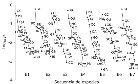
Figura 3. Curvas de rango-abundancia de especies de aves acuáticas que utilizaron los ambientes intermareales de la caleta Malaspina en cada estación de muestreo (E). El número indicado para cada estación corresponde a su ubicación en la figura 1. El código de las especies corresponde al de la tabla 2.
