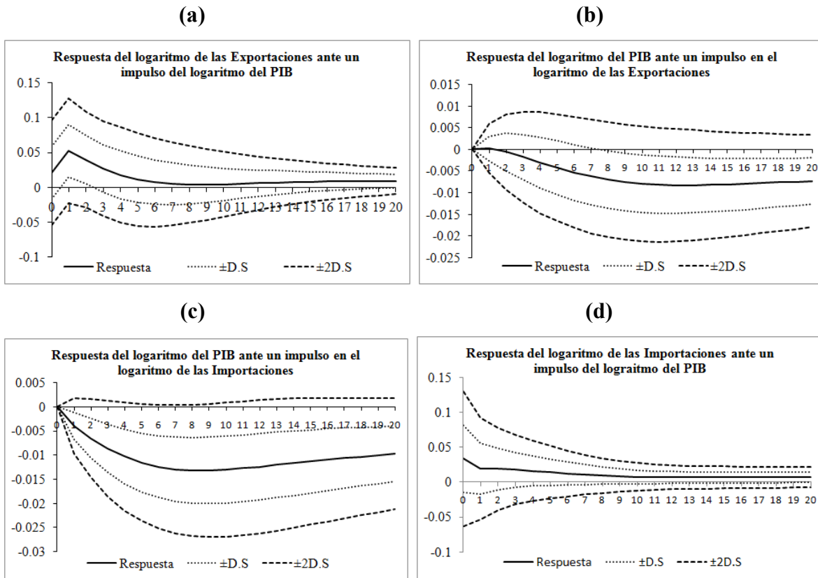
Gráfico 3 Función impulso-respuesta
