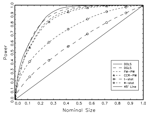
(d) \alpha_1 = 1, \delta = 0.5
