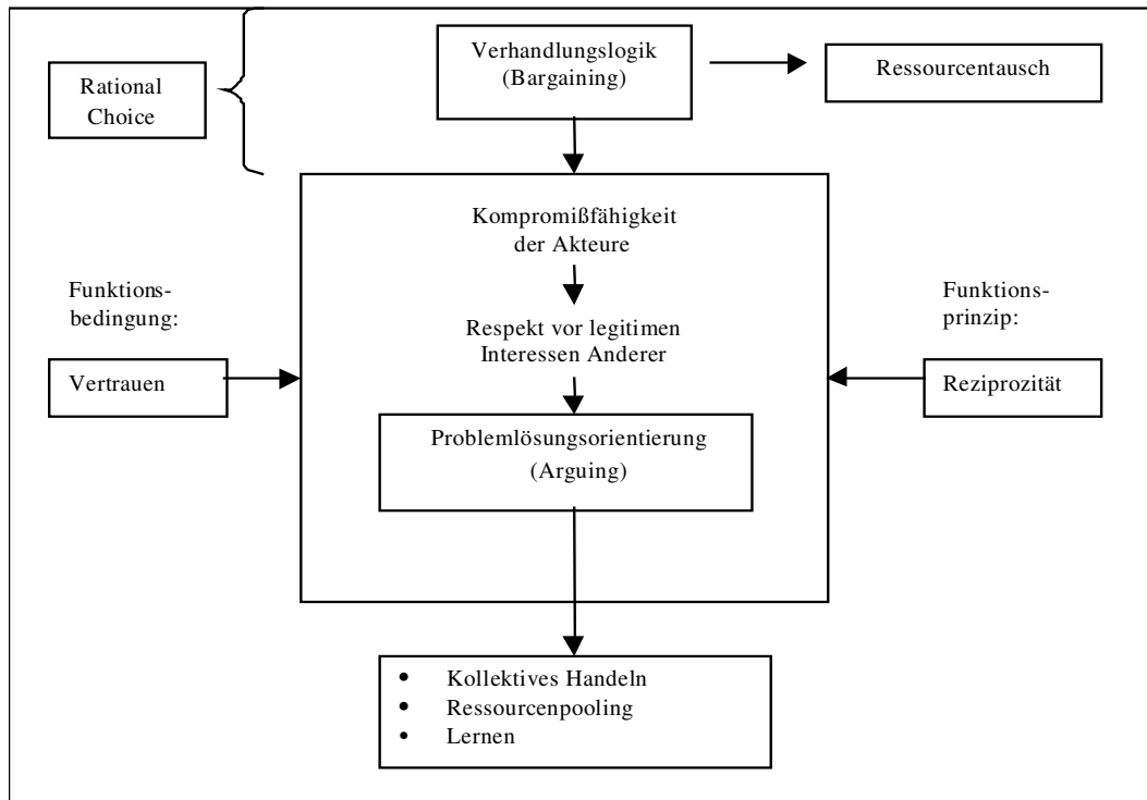
Abbildung 12 Netzwerklogik.
