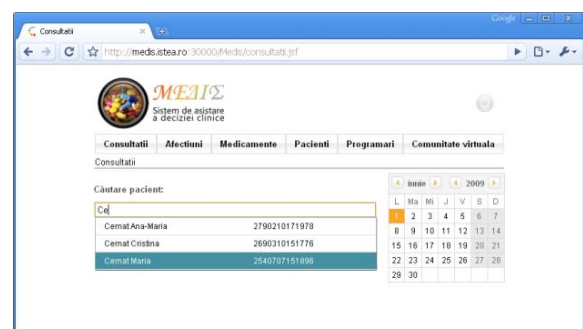
Fig. 5. Search options
