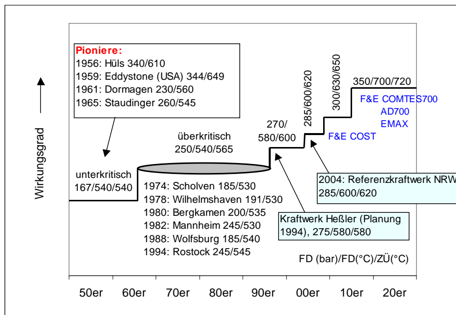
Abbildung 3: Entwicklung von Dampfparametern steinkohlebefuerter Kraftwerke
