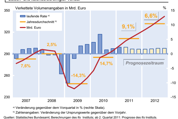
Abb. 4.10 Reale Exporte Saison- und kalenderbereinigter Verlauf
